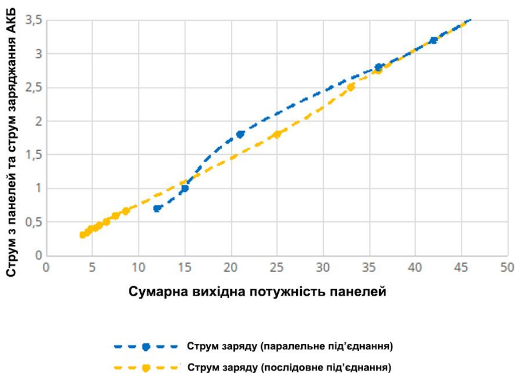
Рис 2.5. Зміна струму при паралельному та послідовному з'єднанні панелей малої потужності у похмуру погоду (фото автора)
