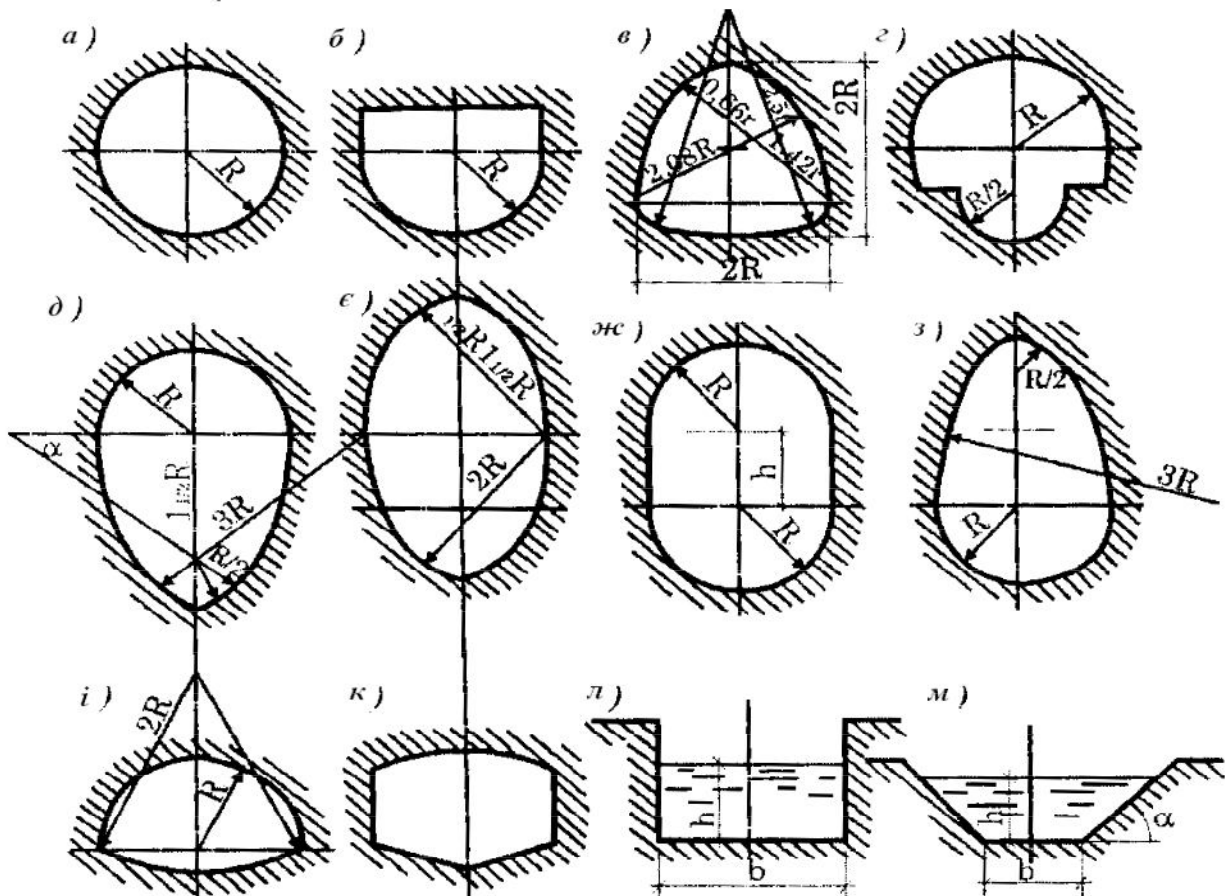
Рисунок 4.4 – Форми поперечного перетину труб і каналів:
