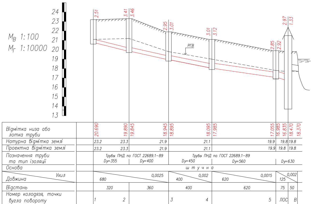
Рисунок 6.4 – Приклад повздовжнього профілю дощового колектора
