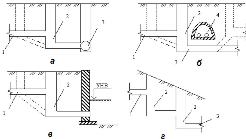
Рисунок 8.8 – Випадки застосування перепадних колодязів: 1 – підвідний трубопровід, 2 – перепадний колодязь, 3 – відвідний трубопровід, 4 – перешкода
