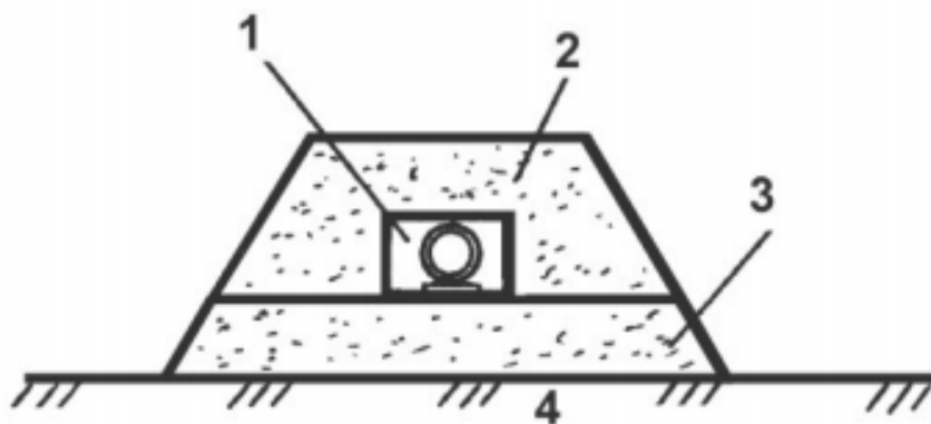
Рисунок 10.2 – Схема наземного прокладання водовідвідних мереж:
