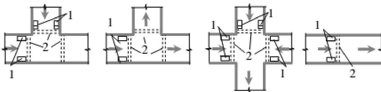
Рисунок 8.7 – Схеми розміщення дощоприймачів на перехрестях та вулицях: 1 – дощоприймачі; 2 – пішохідні переходи
