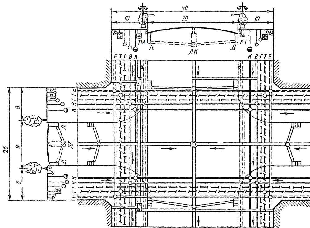
Рисунок 5.1 – Рациональне розміщення підземних мереж:
