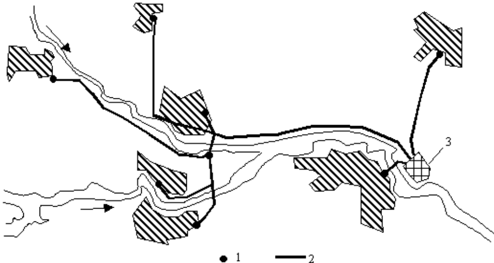
Рисунок 2.13 – Схема групової системи водовідведення: 1 – насосні станції; 2 – магістральні колектори; 3 – очисні споруди
