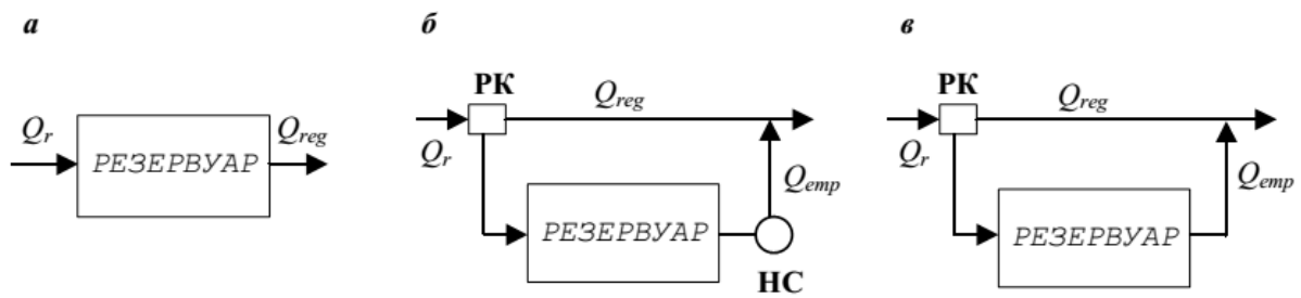
Рисунок 8.14 – Схеми підключення регулюючих резервуарів: РК – розділова камера, НС – насосна станція
