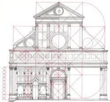
Рисунок 1 – Геометричні пропорції фасаду Санта Марія Новелла
