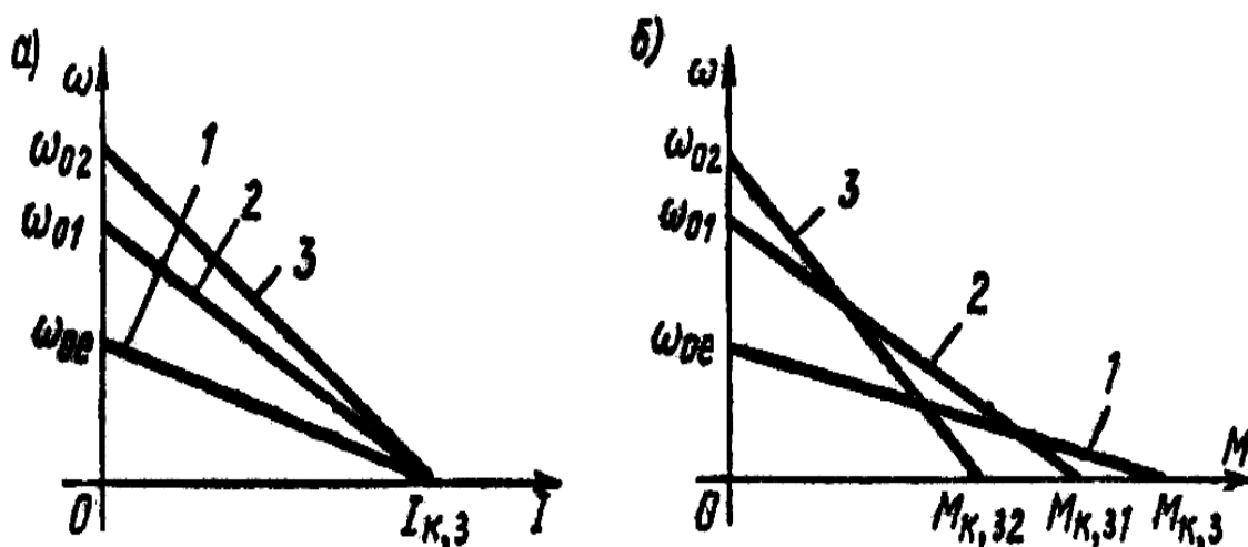
Рисунок 3.15 – Електромеханічні характеристики а) і механічні б) ДПС НЗ при ослаблені збудження
