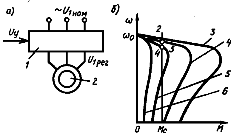
Рисунок 4.14 – Схема регулювання координат АД зміною напруги на статорі (а) і механічні характеристик (б)
