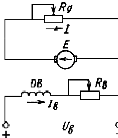
Рисунок 3.7 – Схема динамічного гальмування ДПС НЗ
