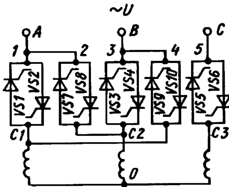
Рисунок 4.17 – Реверсивна схема управління з використанням ТРН
