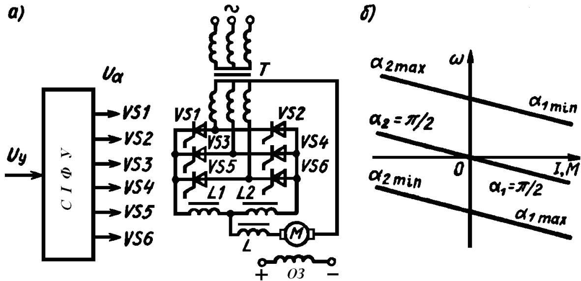
Рисунок 3.20 – Схема ЕП з реверсивним КВ з нульовим виводом (а) і характеристики ДПС НЗ при спільному методі управління тиристорами (б)
