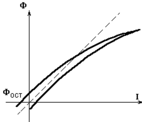
Рисунок 3.22 – Характеристика намагнічення машини постійного струму
