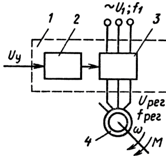
Рисунок 4.21 – Блок схема ПЧ з безпосереднім зв'язком
