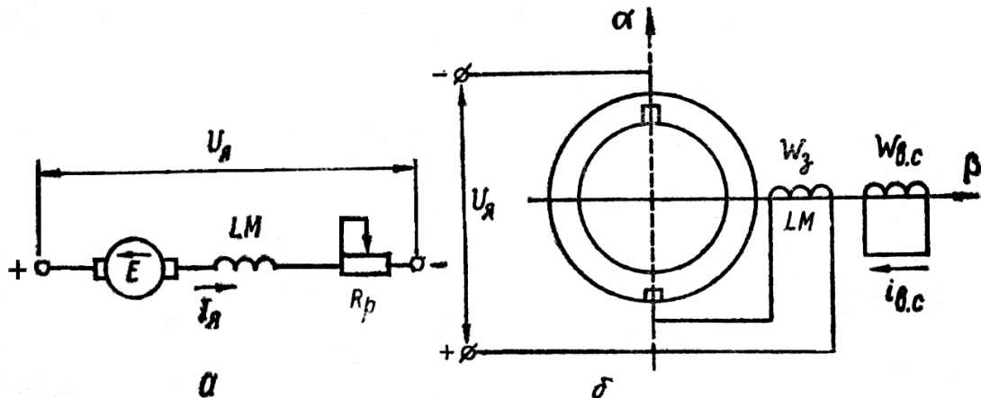
Рисунок 3.21 – Схема двигуна постійного струму послідовного збудження
