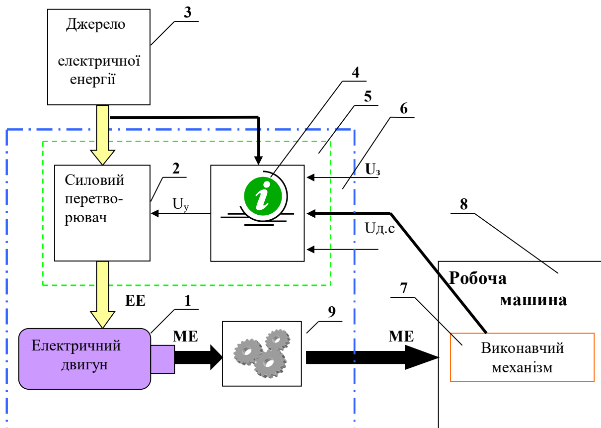
Рисунок 1 – Структурна схема електропривода
