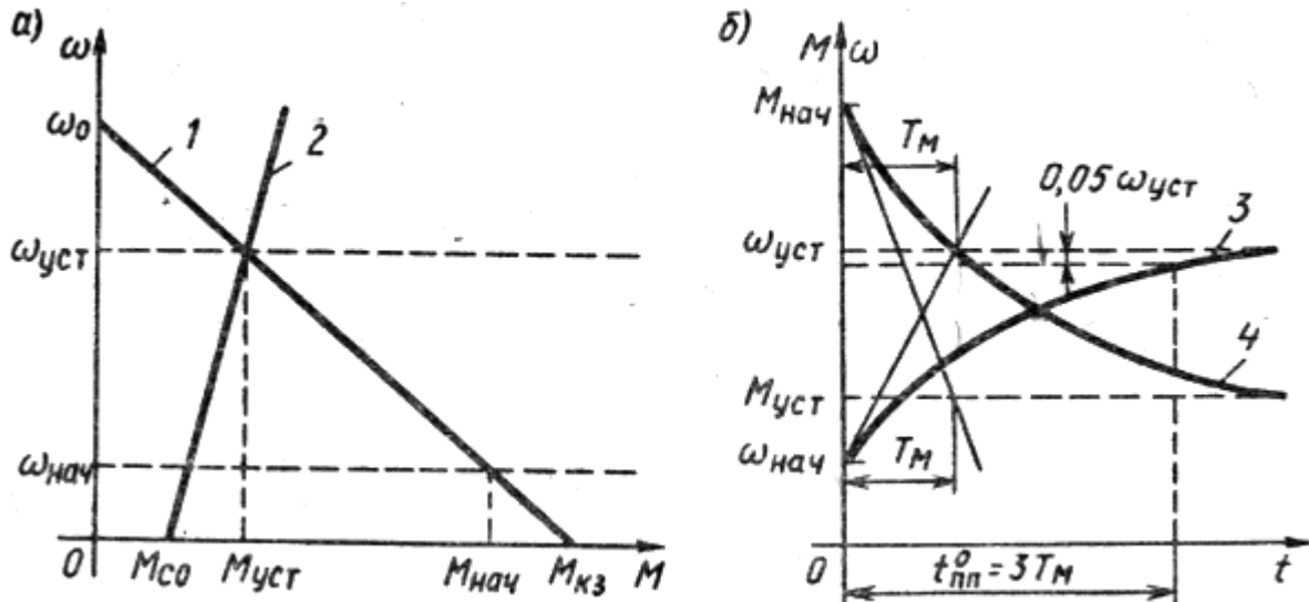
Рисунок 2.9 – Лінійні механічні характеристики двигуна і виконавчого органу (а) і графіки перехідного процесу розгону ЕП (б)
