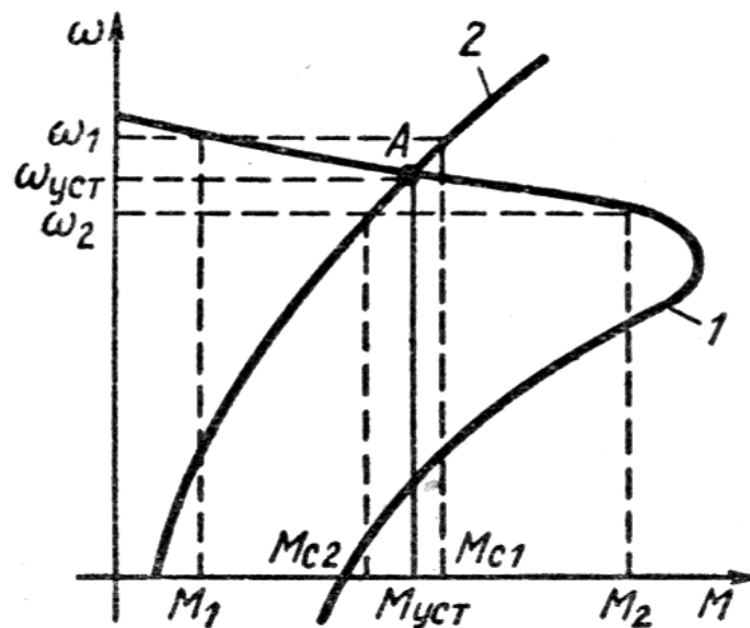
Рисунок 2.7 – Графіки для визначення швидкості усталеного руху і статичної стійкості роботи ЕП
