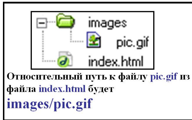
Рисунок 3.13 – Вид записи относительного пути для файлов, находящихся на одном уровне
