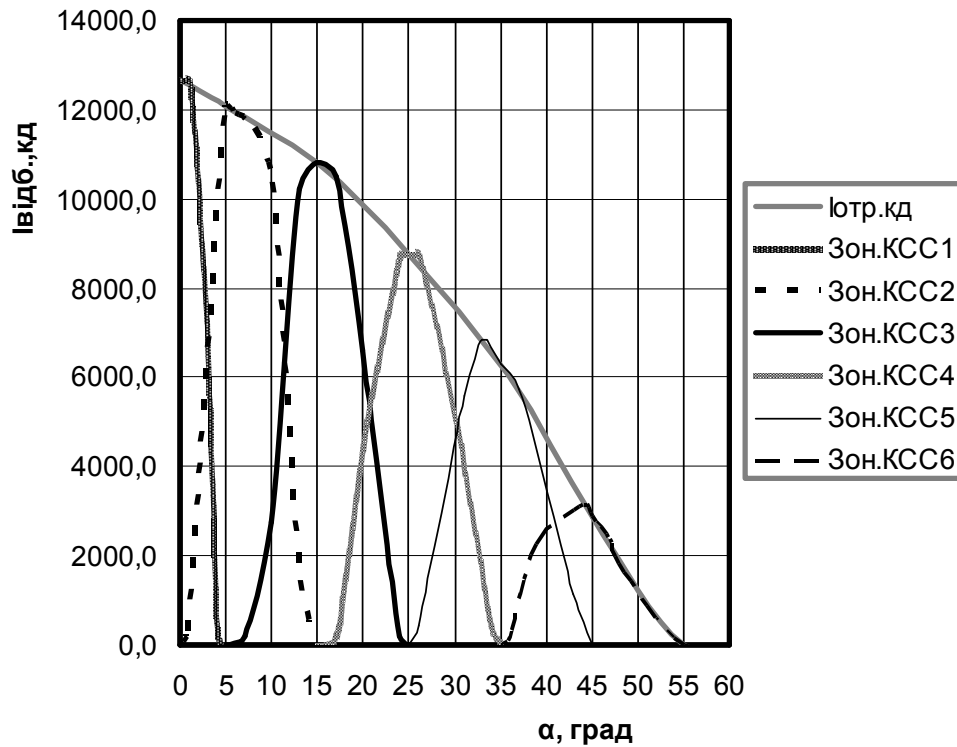
Рисунок 2 – Описання необхідної КСС відбивача зональними КСС
