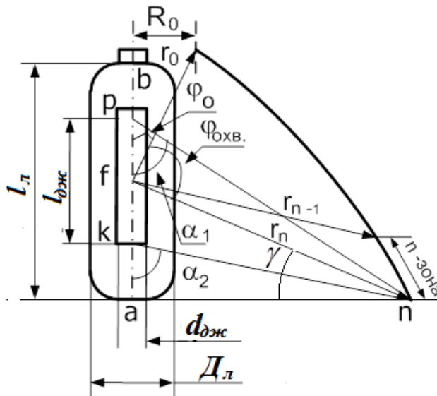
Рисунок 1 – Профіль відбивача СП з заданим світлорозподілом
