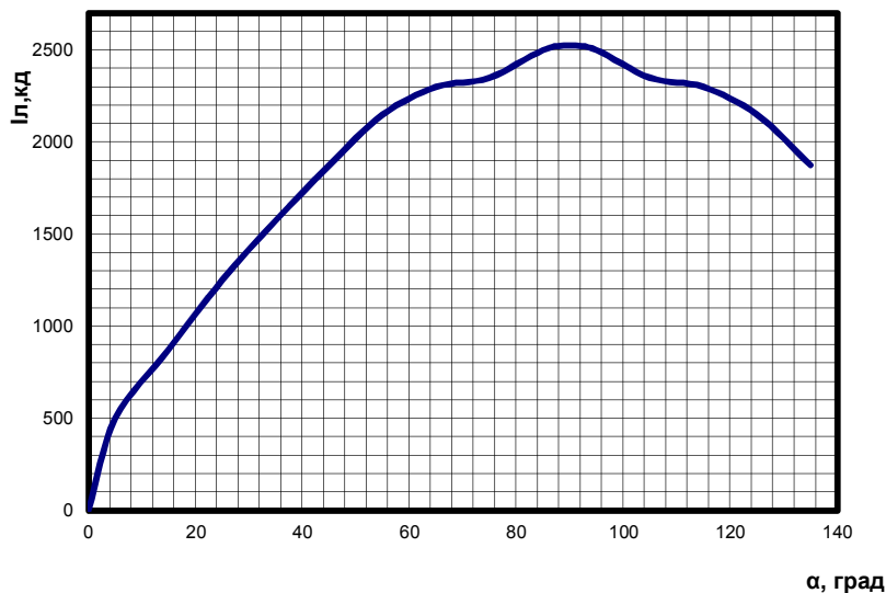
Рисунок 3 – КСС лампи ДНаТ-250
