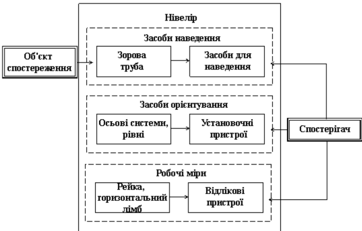
Рисунок 1.3 – Структурна схема нівеліра
