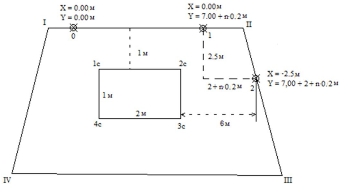
Рисунок 2 – Схема розбивки
