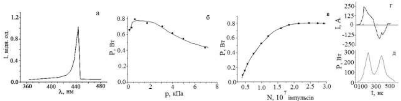
Рис 2. Спектр випромінювання газорозрядної плазми на суміші HgJ_2 : Хе: Не = 100 Па: 1 кПа: 170 кПа а). Залежність середньої потужності випромінювання ексіплексних молекул HgJ^* від парціального тиску ксенону б). Залежність середньої потужності випромінювання ексіплексних молекул HgJ^* від загального числа імпульсів накачування в). г), д). Осцилограми: імпульсів струму розряду і потужності випромінювання відповідно. Суміш HgJ_2 : Хе: Не = 100 Па: 1 кПа: 170 кПа. Амплітуда імпульсів напруги і частота слідування рівні 23 кВ і 18 кГц відповідно.
