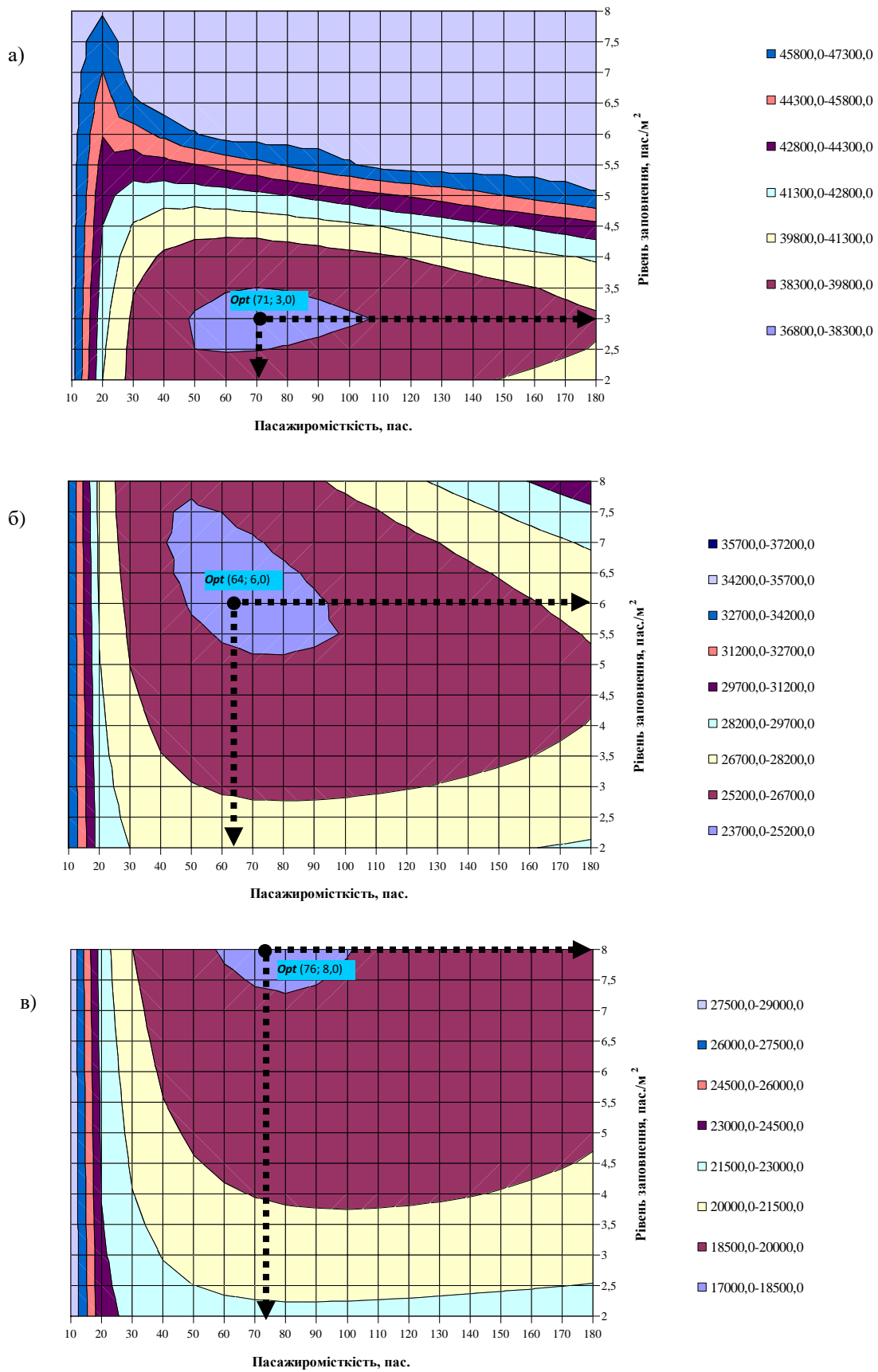
Рис. 1. Контурні діаграми зміни сукупних витрат за F_{\text{max}} = 720 пас./год та наступних значень коефіцієнту нерівномірності пасажиропотоку за довжиною маршруту:
