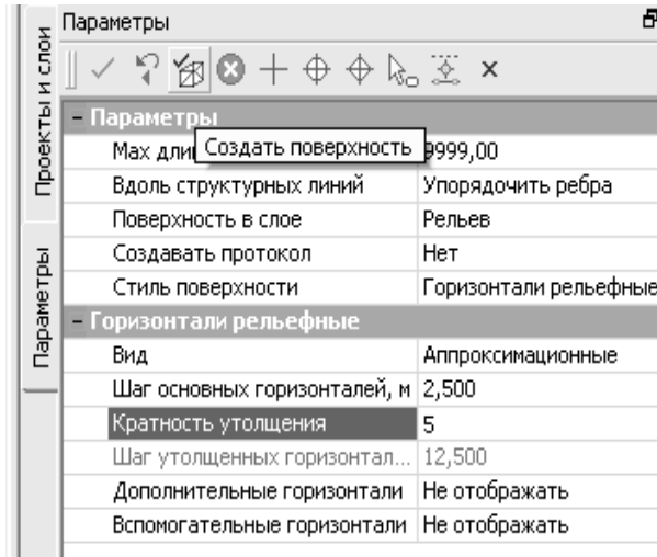
Рис. 3. Параметри побудови поверхні
