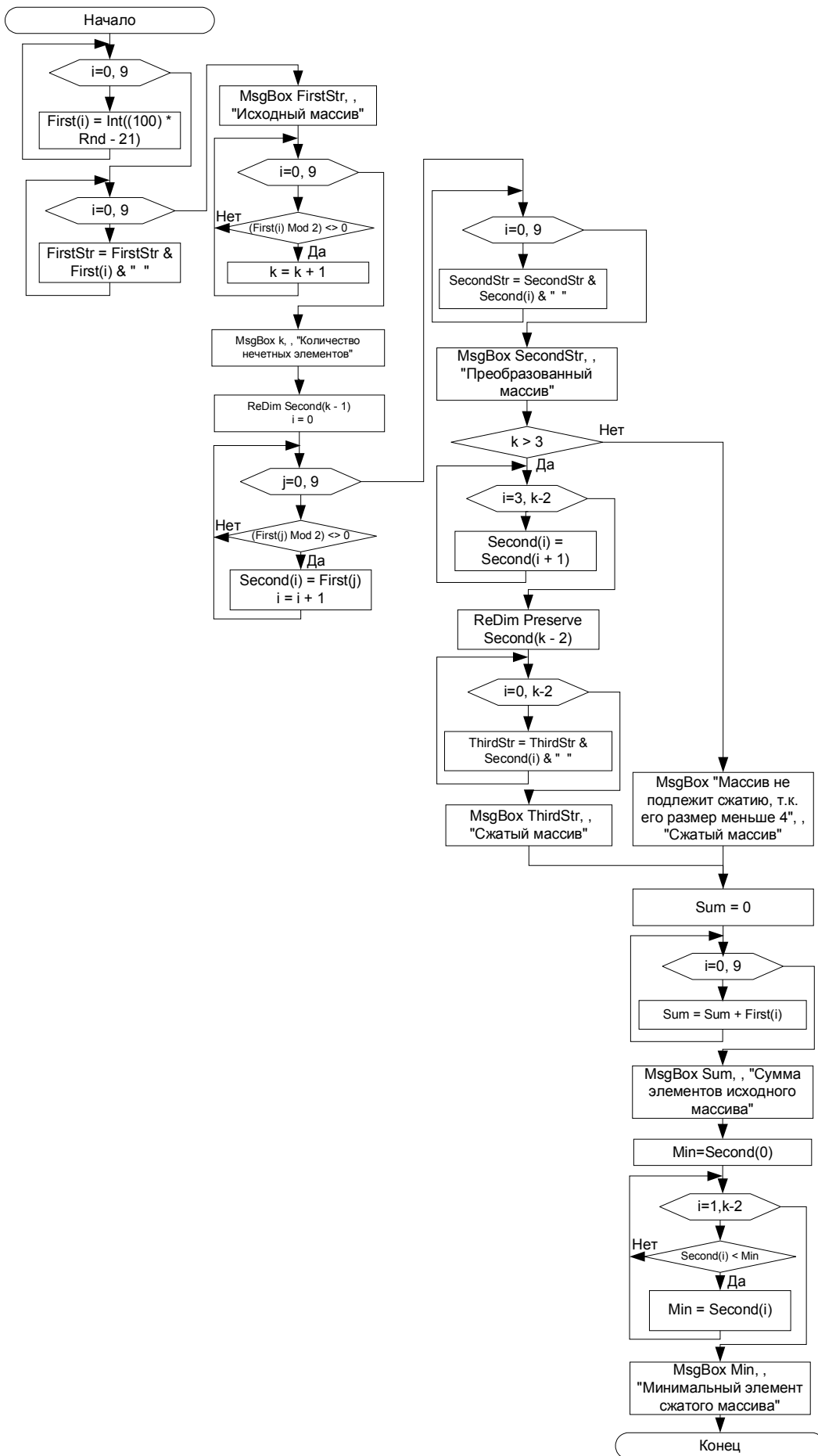
Рисунок 2 – Блок схема алгоритму
