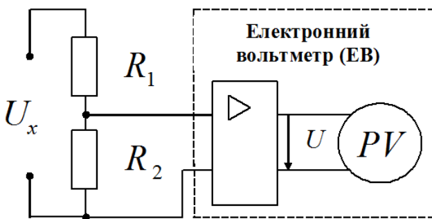
Рисунок 4.5 – Схема вимірювання напруги
