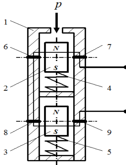
Рисунок 7.2 – Датчик тиску з віброкомпенсацією (патент України № 102622):
