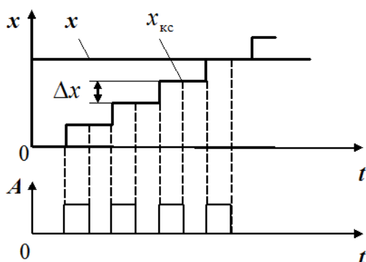
Рисунок 4.9 – ЦВП число-імпульсного квантування
