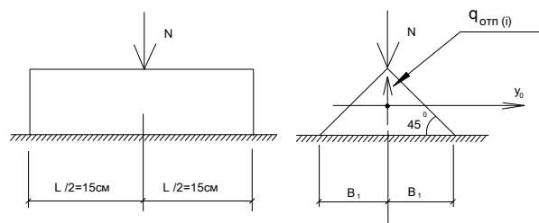
Рис. 3. Розрахункова схема
