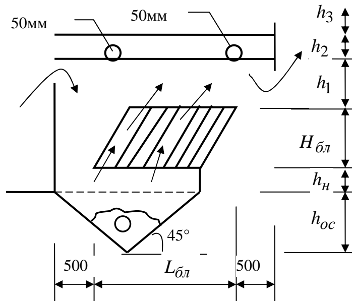
Рис.2 - Схема відстійного відділення
