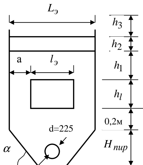
Рис.1 - Схема электродної камери
