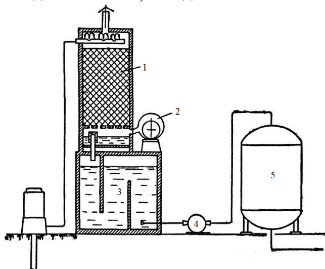
Рисунок 3.1 – Схема установки для знезалізнення води аерацією: 1 – вентиляторна градирня; 2 – вентилятор; 3 – контрактний резервуар; 4 – насос; 5 – фільтр
