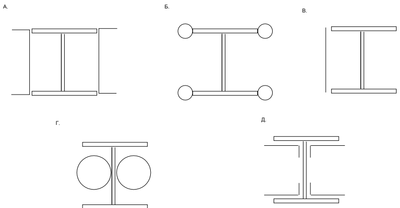
Рисунок 1 - Схеми підсилення колон
