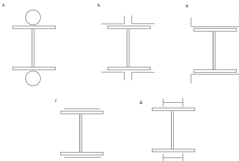
Рисунок 2 - Схеми підсилення головних балок
