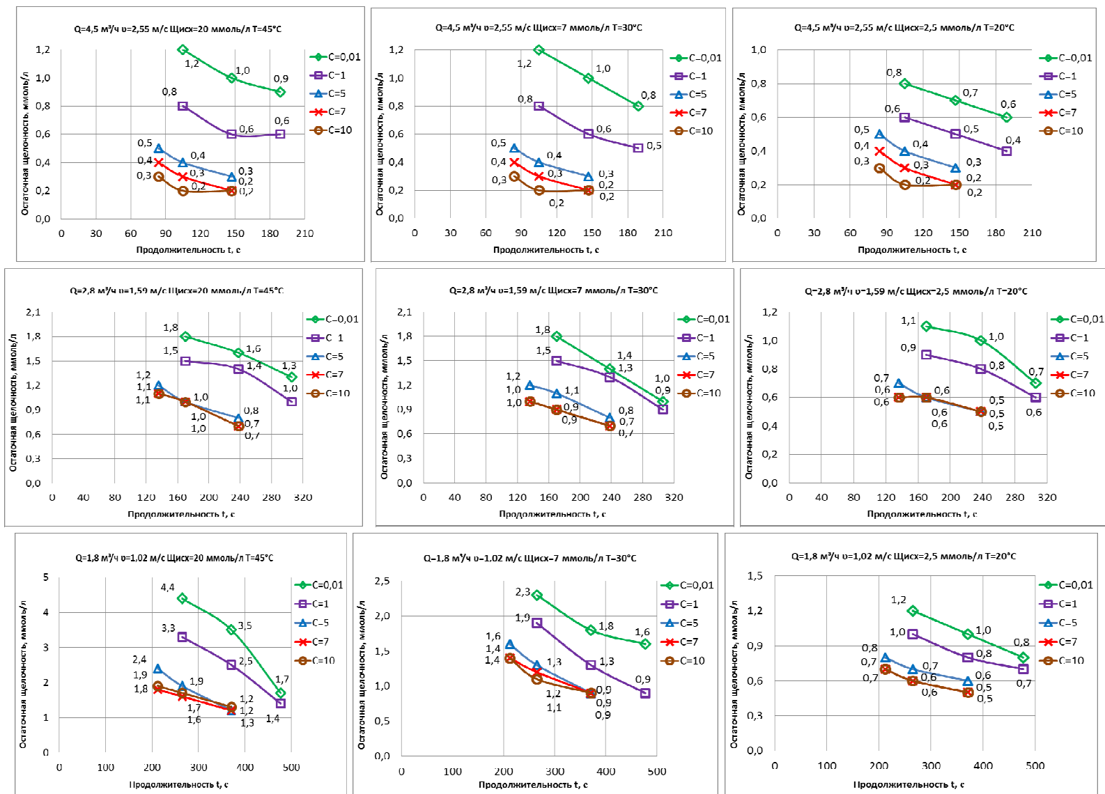
Рисунок 1 – Графики зависимости остаточной щелочности (ОЦ) от продолжительности перемешивания (t) после модернизированного аппарата D=150 мм L= 1500 мм в промышленных условиях при интенсивном перемешивании воды с содержанием масел 25-35 мг/л
