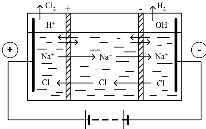
Рисунок 6.12 – Схема трикамерної електродіалізнаї ванни
