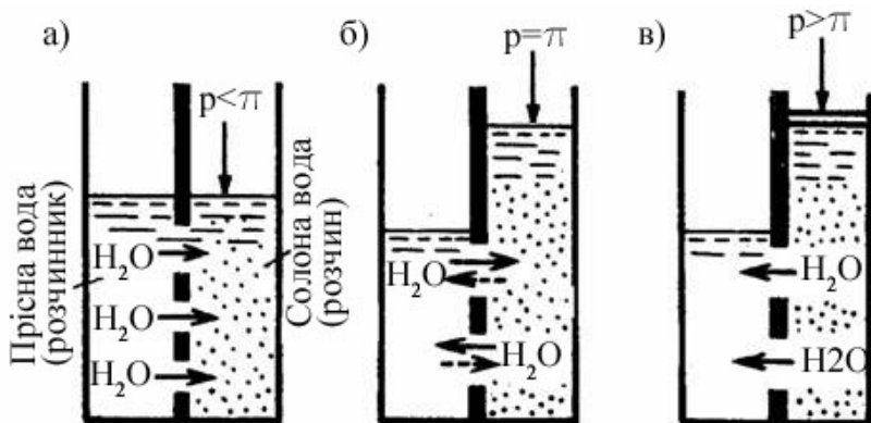
Рисунок 6.15 – Схема виникнення зворотнього осмосу: а – осмос; б – рівновага; в – зворотній осмос
