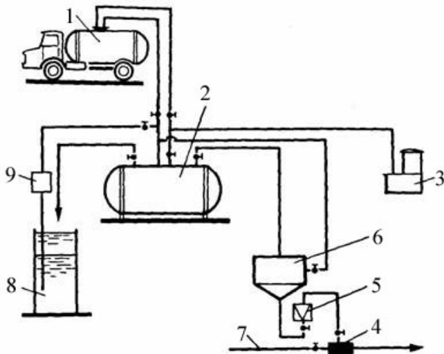
Рисунок 3.3 – Фтораторная установка з використанням кремнефтористоводневої кислоти:
