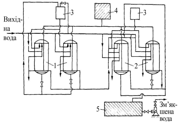
Рисунок 2.3 – Схема двоступінчастого Na-катіонітового зм'якшення води:
