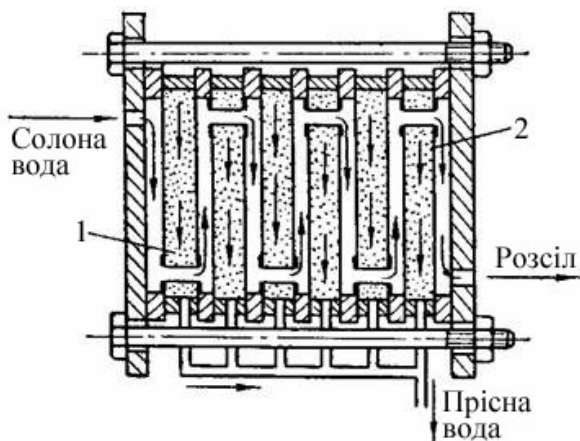
Рисунок 6.15– Схема зворотньоосмотичного апарату з плоскокамерними елементами:
