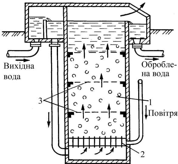
Рисунок 5.1 – Аератор
