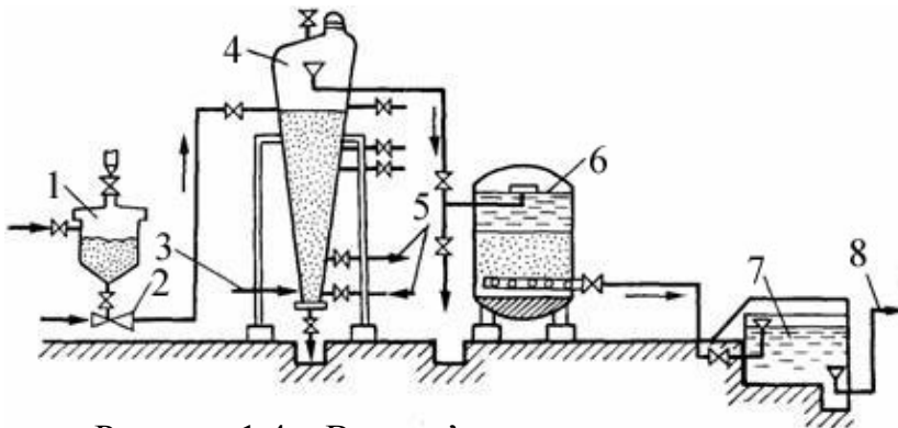
Рисунок 1.4 – Водозм'якшувальна установка з вихровим реактором:
