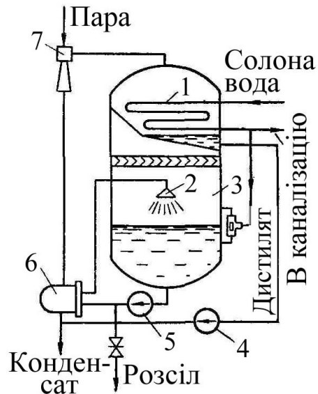
Рисунок 6.4 – Одноступінчастий адіабатний випарник:
