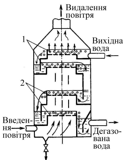
Рисунок 5.5 – Схема дегазатора пінного типу: 1 – пінний шар; 2 – дірчасте днище
