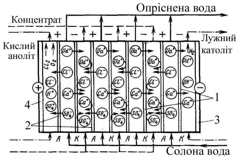
Рисунок 6.13 – Схема багатоканального електродіалізного апарату:
