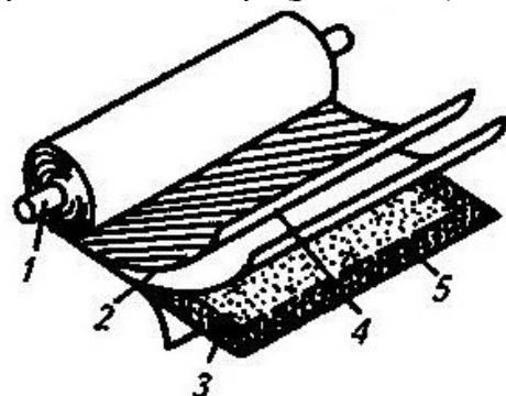
Рисунок 6.16 – Рулонний елемент в розмотаному вигляді:
