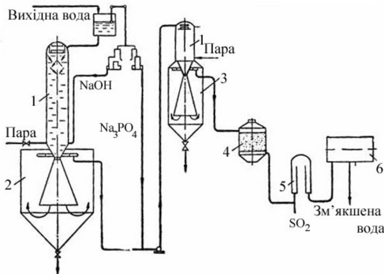
Рисунок 1.5 – Схема термохімічної установки з фосфатним дозм'якшенням:
