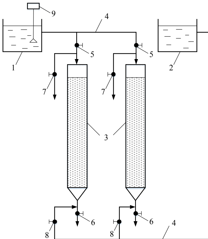
Рисунок 3.4 – Установка для дослідження процесу фільтрування: 1 – бак вихідної води; 2 – бак промивної води; 3 – фільтрувальні колонки; 4 – трубопроводи; 5 – крани подавання вихідної води; 6 – крани для збирання фільтрату; 7 – крани для збирання промивної води; 8 – крани для подавання промивної води; 9 – електрична мішалка
