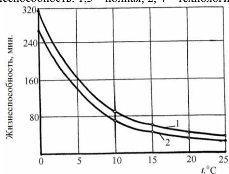
Рис. 3. Зависимость жизнеспособности клея от температуры окружающей среды. Жизнеспособность: 1 – полная, 2 – технологическая
