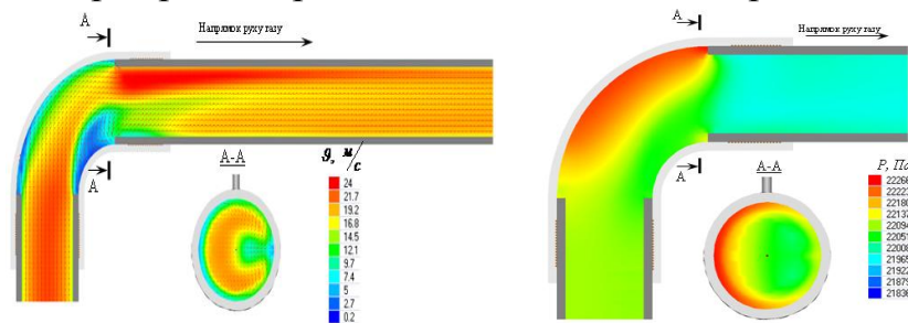
Рис. 1 – Розподіл модуля швидкості потоку газу, вектори швидкості газу та розподіл тиску в площині горизонтального повздовжнього перерізу терморезисторного коліна
