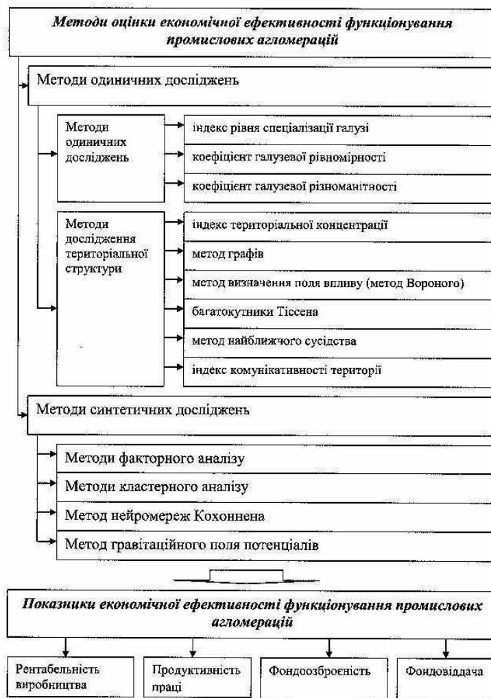
Рис. 1. Методи суспільно-географічного дослідження промислових агломерацій
