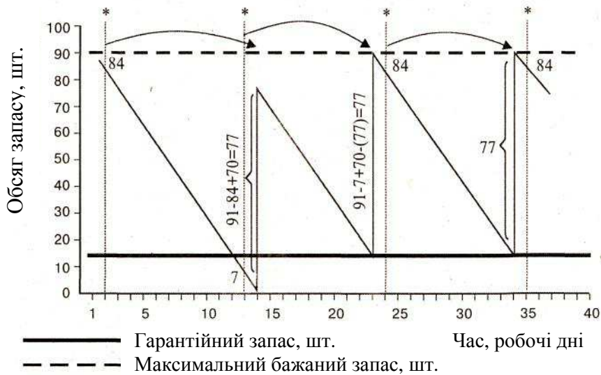
Рис. 3.2 – Графічна модель роботи системи управління запасами з фіксованим інтервалом часу між замовленнями при наявності однієї затримки у поставках
