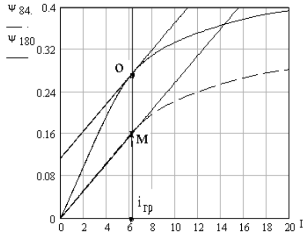
Рис. 3. Параллельный перенос участка кривой намагничивания от линии граничного тока до максимального тока в согласованном положении ротора на кривую при рассогласованном положении ротора
