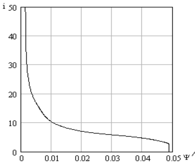
Рис.2. Зависимость тока от производной от потокоцепления по току (динамической индуктивности)
