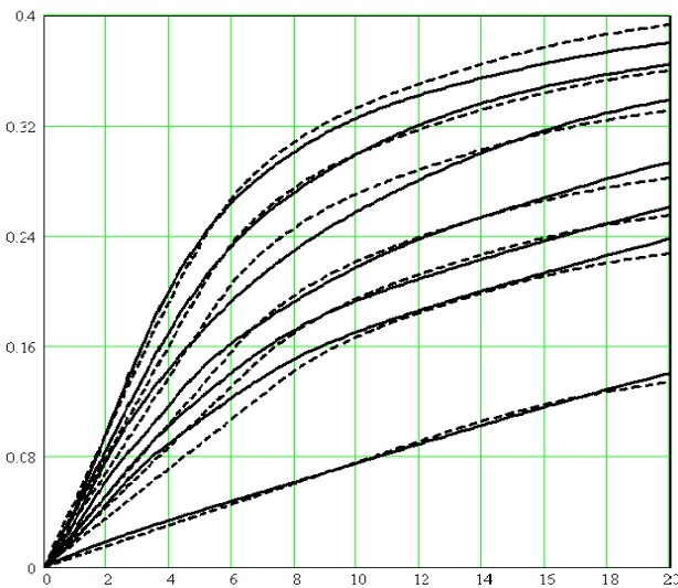
Рис.1 Семейство кривых намагничивания ВИРД \Psi(i, \zeta) при углах поворота ротора 180, 126, 108, 84, 72, 60 и 0 электрических градусов (сплошные линии – экспериментальные кривые, штриховые – расчетные)
