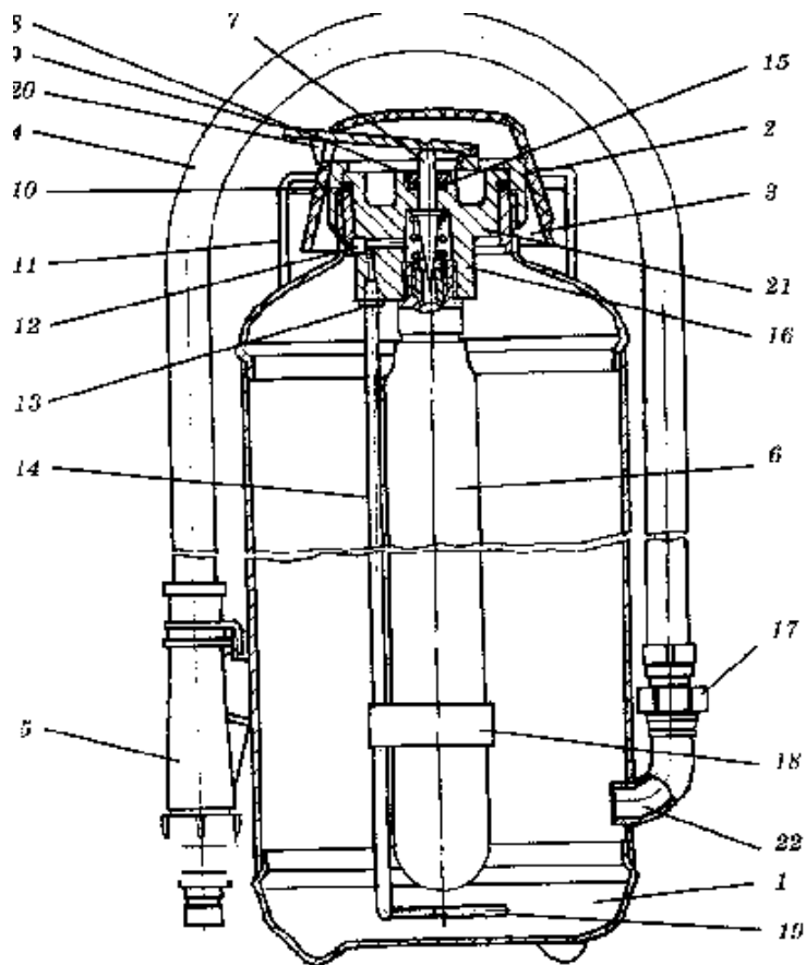
Рис. 8.4 – Вогнегасник порошковий ОП-5.01
