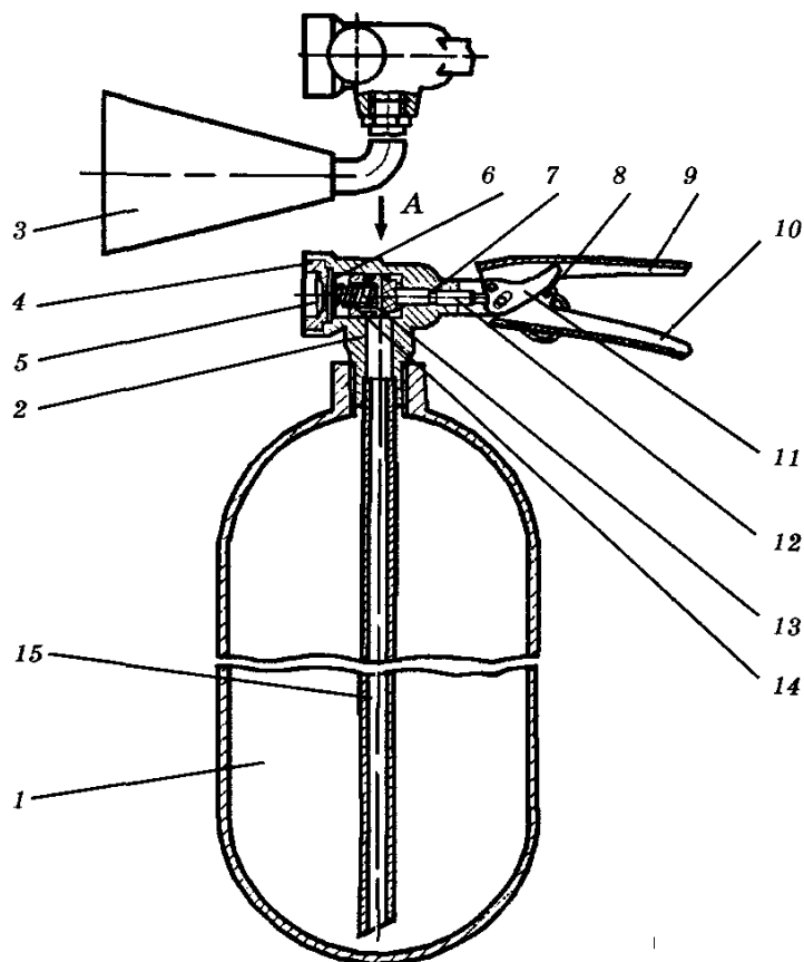
Рис. 8.3 – Вогнегасники вуглекислотні ОВ-2 (ВВК-1,4); ОВ-5 (ВВК3,5): 1 – корпус; 2 – голівка; 3 – розтруб; 4 – гайка; 5 – запобіжна мембрана; 6 – шайба; 7 – кільце ущільнювальне; 8 – запобіжна чека; 9 – важіль керування клапаном; 10 – ручка; 11 – кулачок; 12 – шток; 13 – клапан; 14 – пружина; 15 – трубка сифонна
