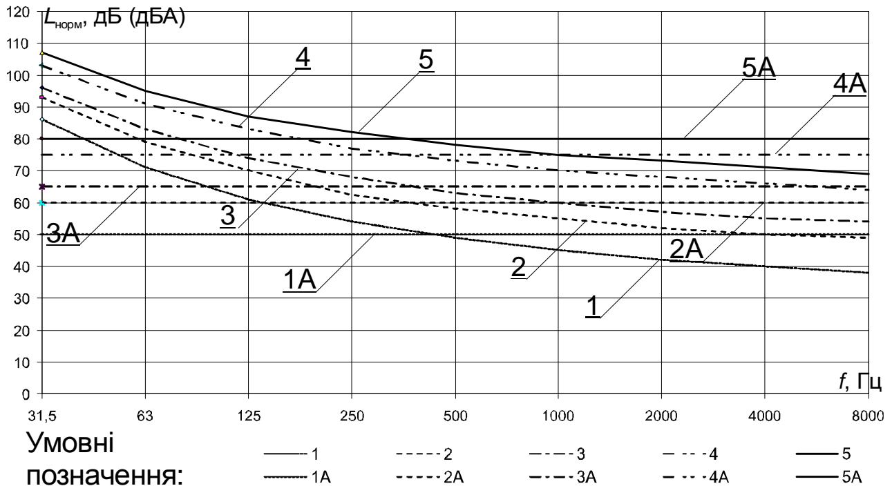
Рис. 3.1 – Нормативні спектри шуму (рівні звуку та звукового тиску згідно з ДСН 3.3.6.037-99 для різних видів діяльності):
