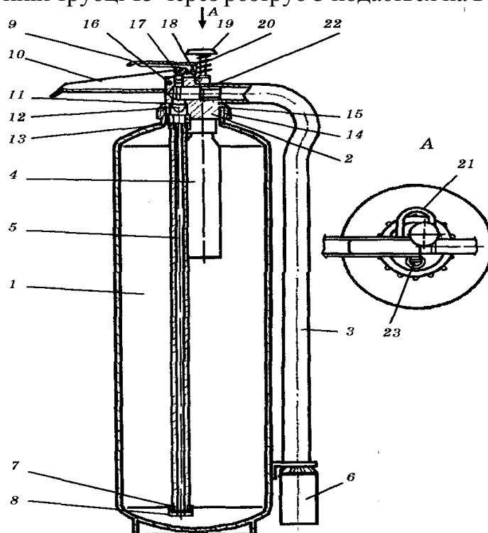
Рис. 8.2 – Вогнегасник повітряно-пінний ОВП-9:
