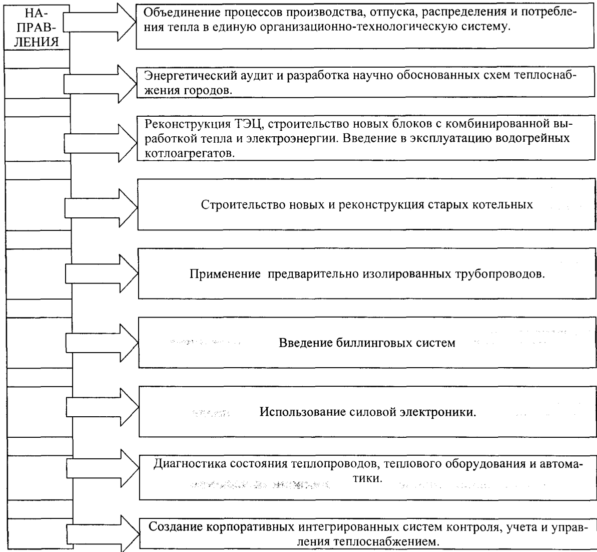
Рисунок 1 – Основные направления повышения эффективности систем теплоснабжения
