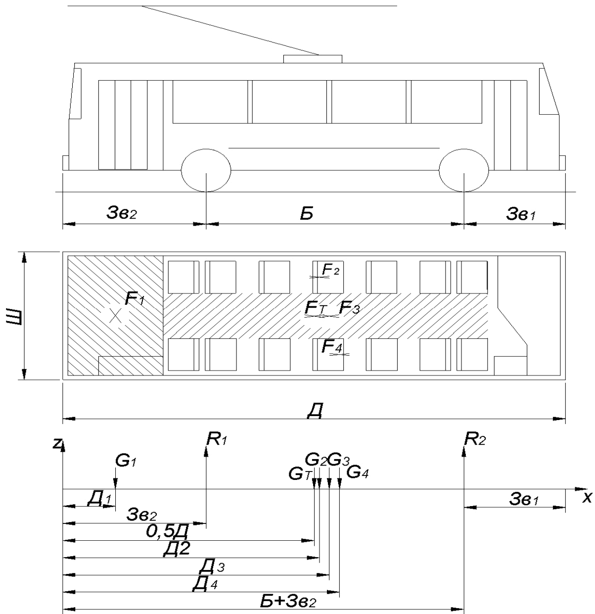
Рис. 3.1 – Вагові навантаження на мости двовісного тролейбуса
