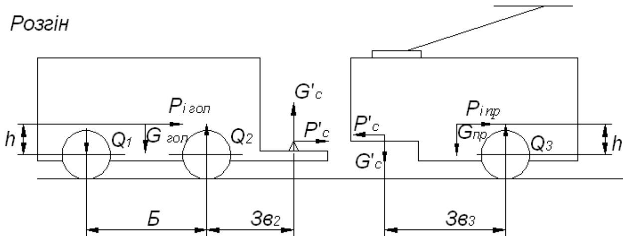
Рис. 8.2 – Додаткові вертикальні й горизонтальні навантаження при гальмуванні й пуску шарнірно-з'єднаних тривісних тролейбусів
