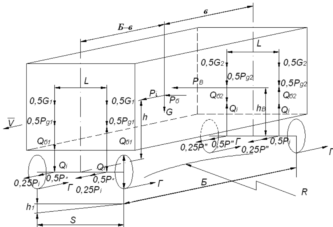
Рис. 9.1 – Схема сил при розрахунку двовісного тролейбуса (гальмування)
