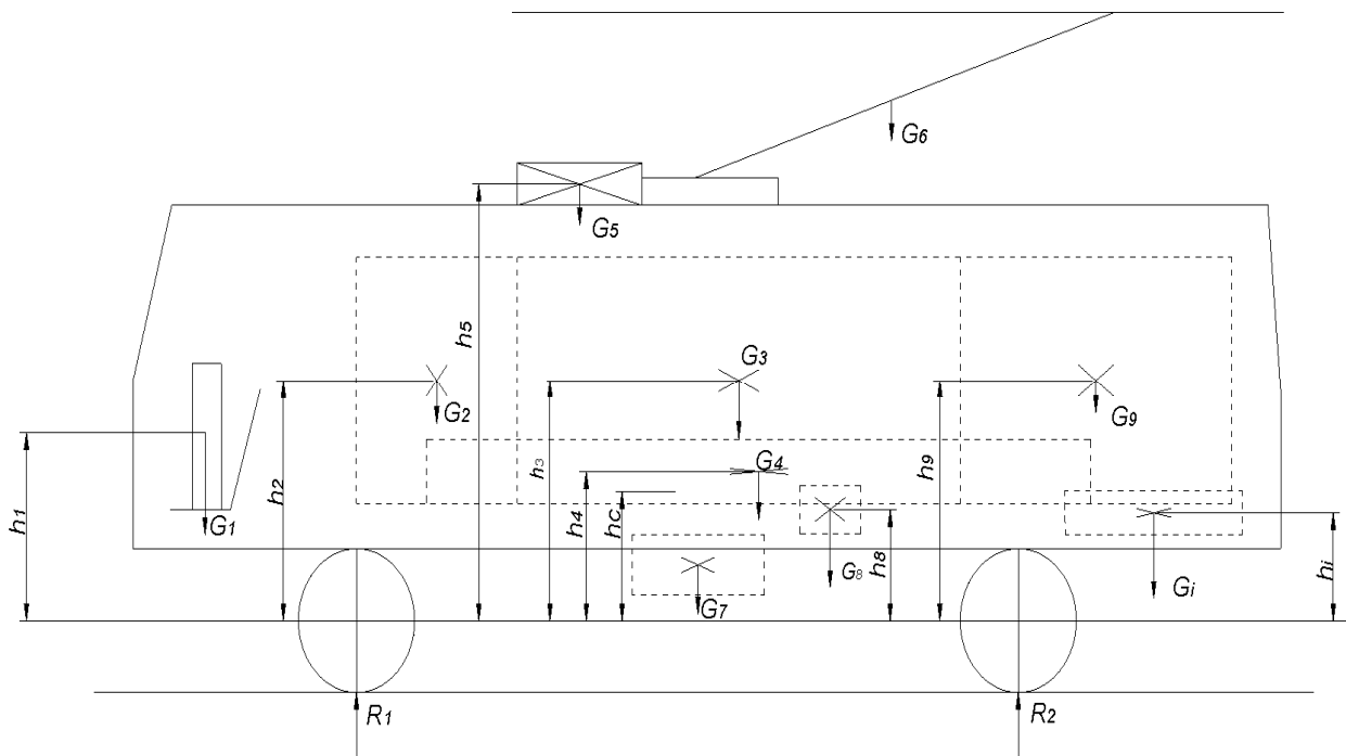
Рис. 4.1 – Схема до визначення центра ваги рухомого складу
