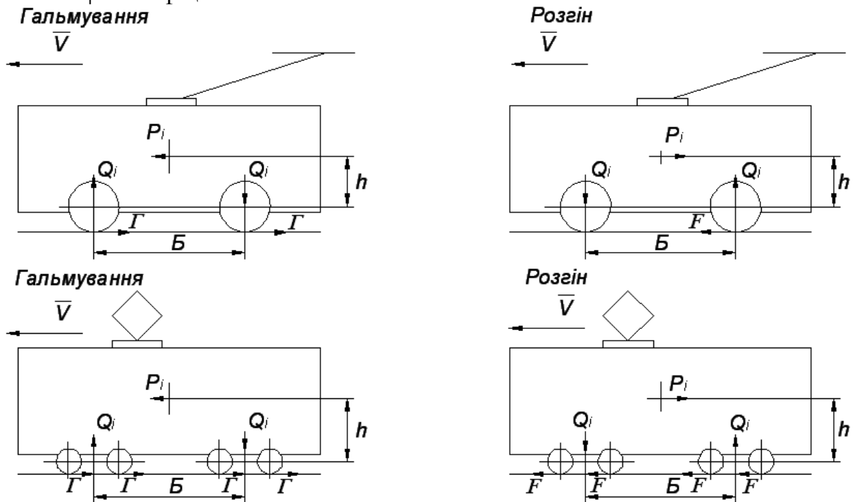
Рис. 8.1 – Додаткові вертикальні й горизонтальні навантаження тролейбуса і трамвая при гальмуванні й пуску
