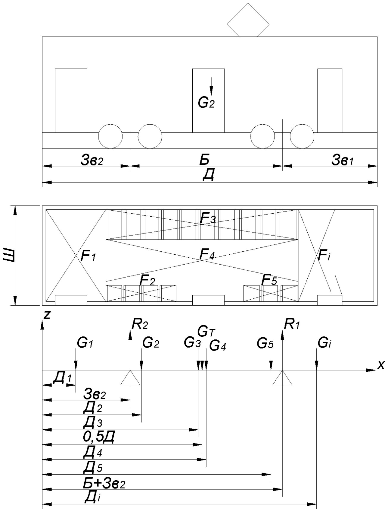
Рис. 3.2 – Вагові навантаження на візки чотиривісного трамвайного вагона
