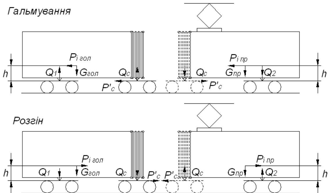
Рис. 8.3 – Додаткові вертикальні й горизонтальні навантаження при гальмуванні й пуску шарнірно-з'єднаних трамваїв
