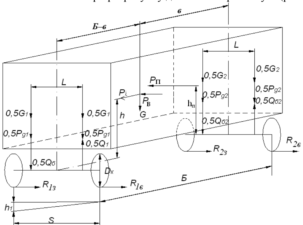
Рис. 9.2 – Схема сил при розрахунку двовісного тролейбуса (розгін)
