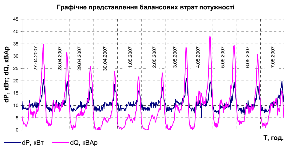
Рис. 1 – Приклад графіку зміни балансових втрат потужності у МЕМ
