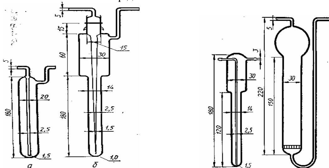
Рис. 2 – Поглинальні прилади:
