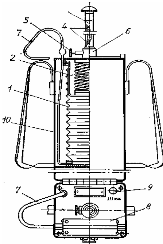
Рис. 3 - Пристрій універсального газоаналізатора типу УГ-2:
