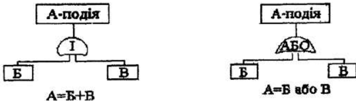
Рис. 3.1 — Логічні операції
