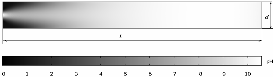
Рис. 2 - Розподіл активної реакції середовища рН в об'ємі трубчастого змішувача-реактора
