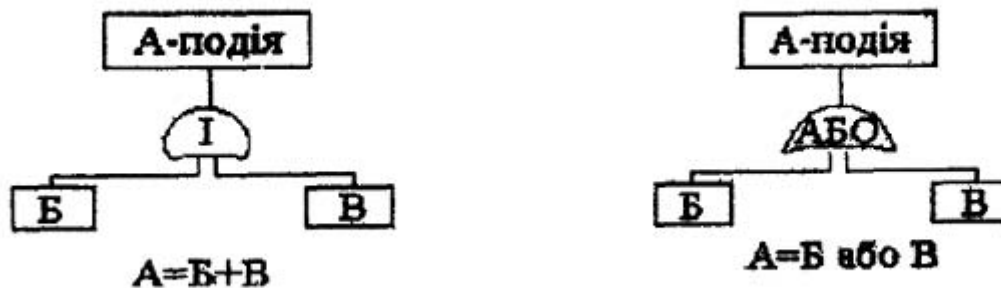
Рис. 3.1 — Логічні операції
