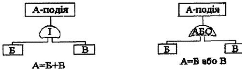
Рис. 3.1 — Логічні операції
