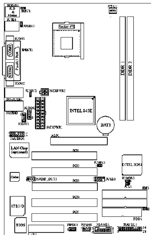
Рис. 1.4 – МП формату АТХ з рознімачем Socket-478
