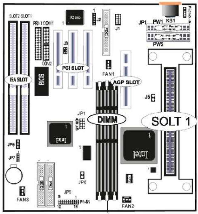
Рис. 1.2 – МП формату mini-AT с різніачем Slot-1
