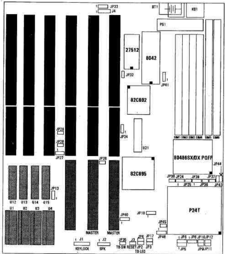
Рис. 1.1 – МП формату 3/4 Baby-AT з різніачем Socket-3
