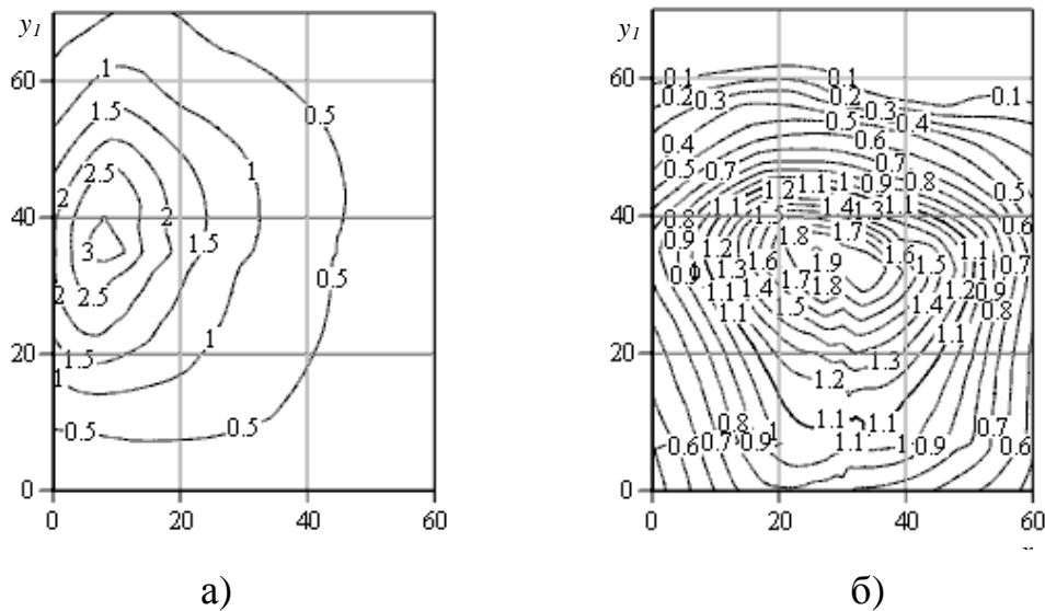
Рис. 1 – Криві однакового опромінення ФАР від опромінювача РСП-ВОТ-02 з ДНаТ-400 ( h=3 м, \zeta_0=60^\circ ): горизонтальної площини – а); вертикальної площини – б)
