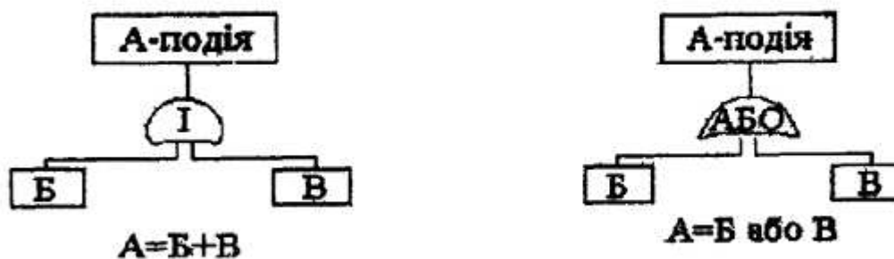
Рис. 3.1 — Логічні операції
