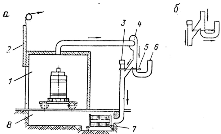
Рис. 11.1 – Схема електричної печі для сушіння обмоток електричних машин
