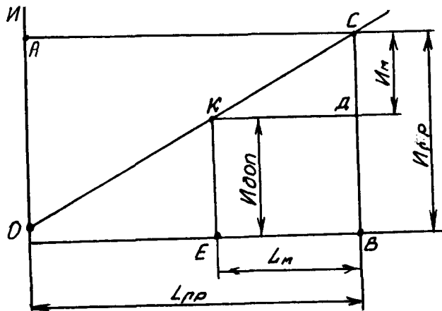
Рис. 6.1 – Визначення допустимого зносу
