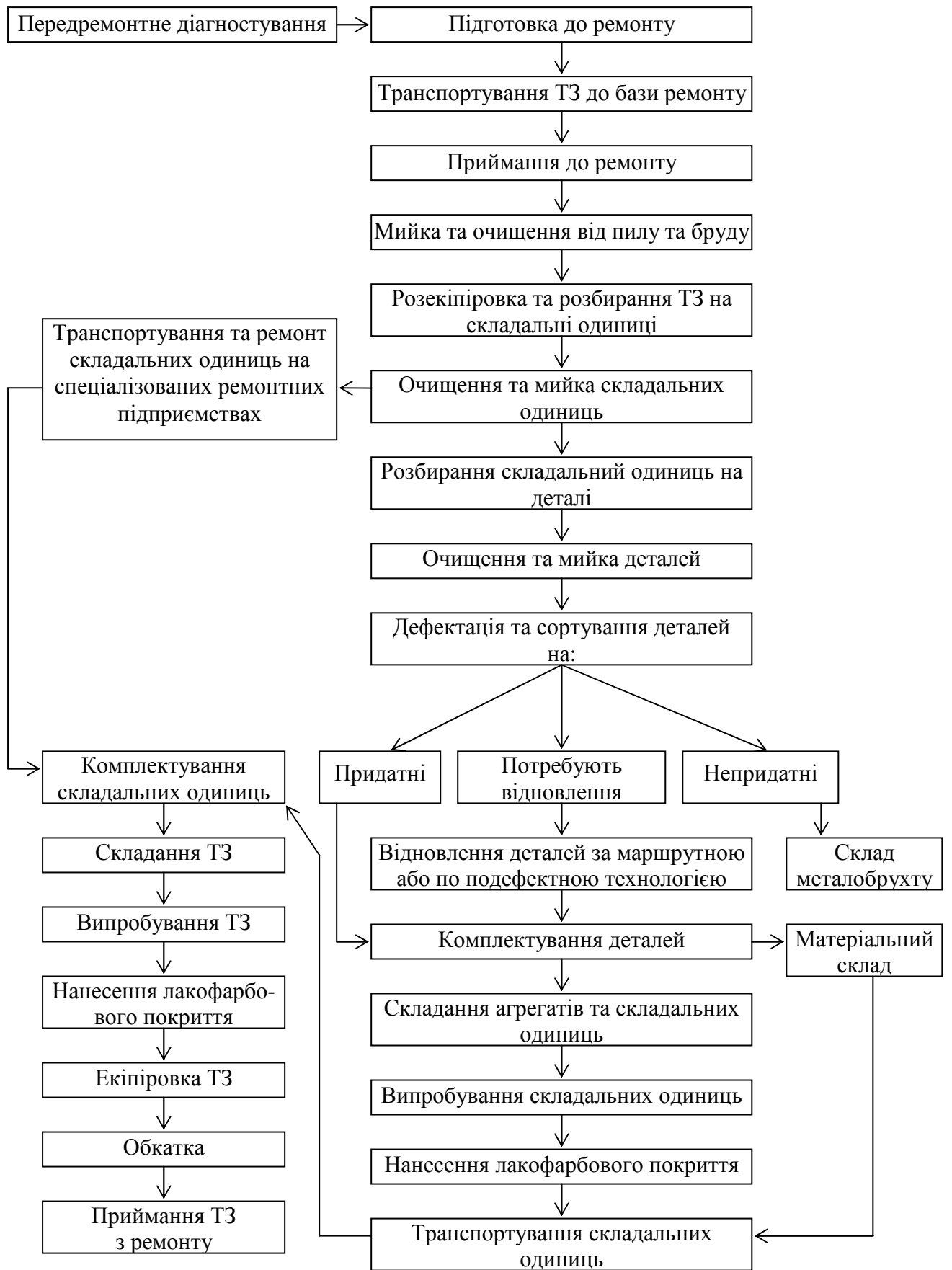
Рис. 3.1 – Блок-схема виробничого процесу ремонту транспортних засобів
