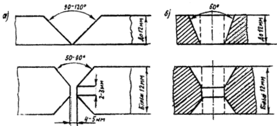
Рис. 9.1 – Підготовка тріщини (а) і отвору (б) до зварювання
