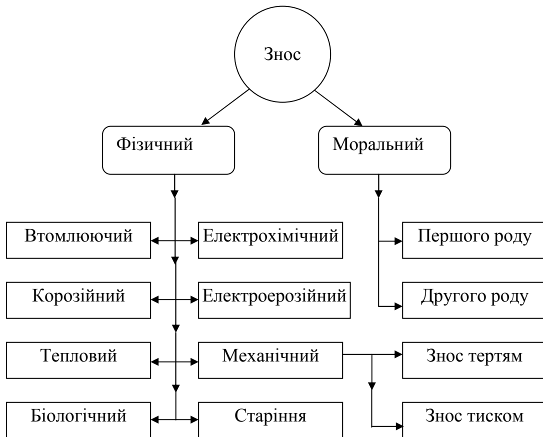
Рис. 1.2 – Види зносу
