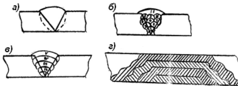
Рис. 9.2 – Схема наповнення шва під час зварювання залежно від його розмірів: а) прохідного; б) багатопрохідного; в) багат шарового; г) методом "гірки"
