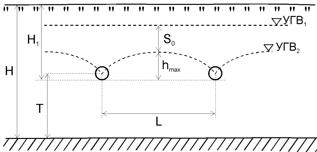
Рис. 1.3 Горизонтальний систематичний дренаж недосконалого типу
