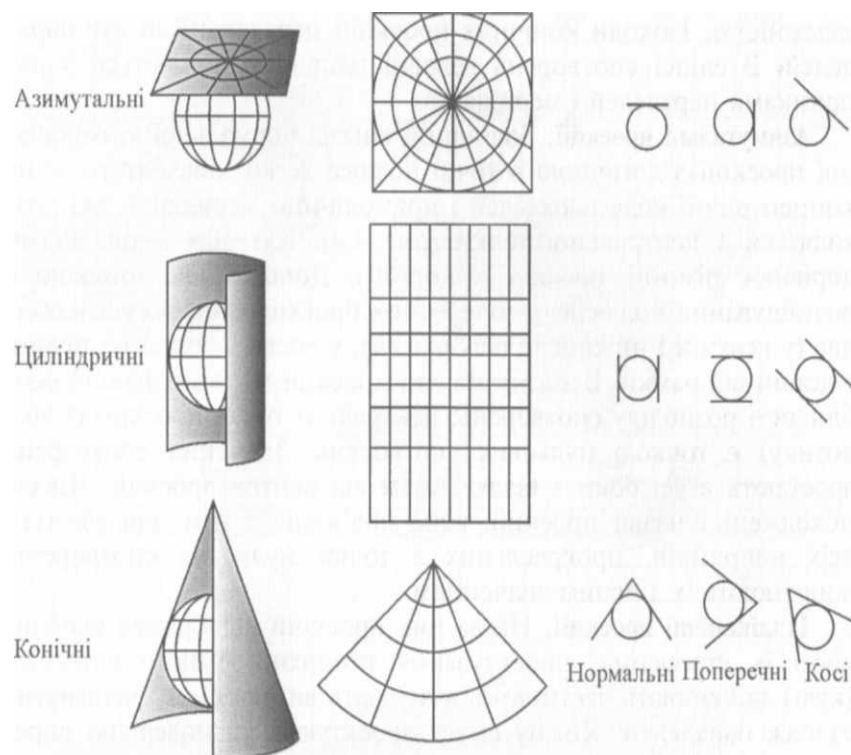
Рис.3.1.– Картографічні проекції:
