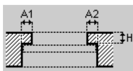
Эскиз проема с определением параметров четверти
