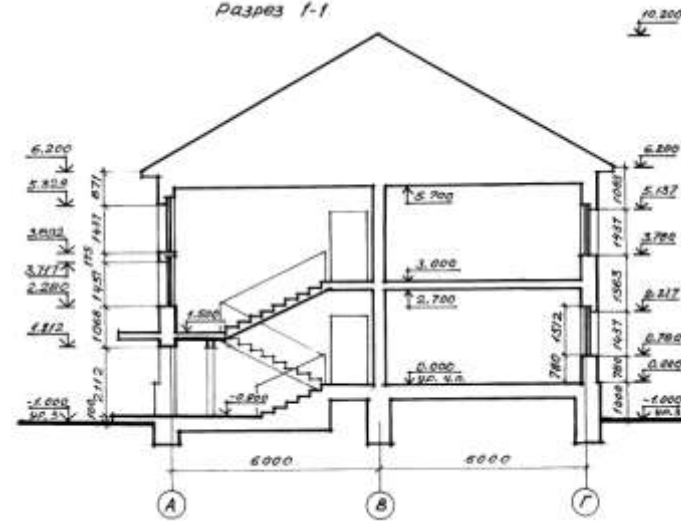
Разрез 1-1
