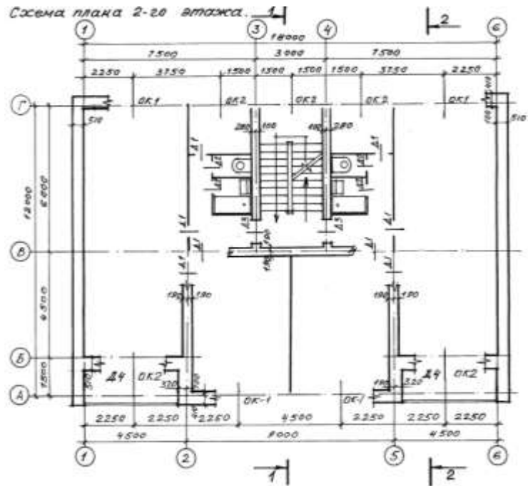
Схема плана 2-го этажа
