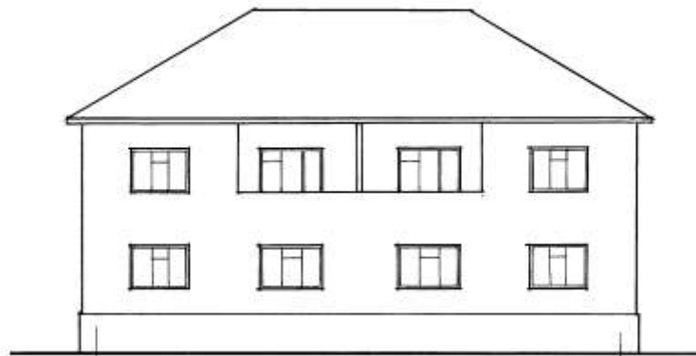
Фасад 1-6
