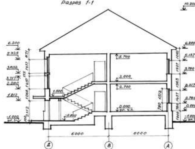
Разрез 1-1
