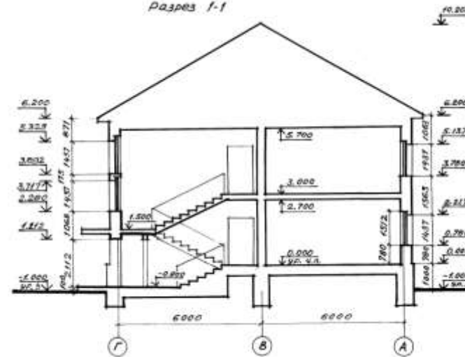
Разрез 1-1
