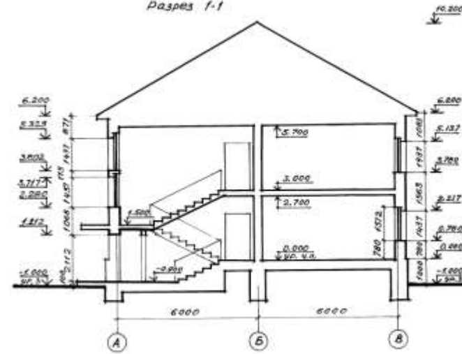
Разрез 1-1
