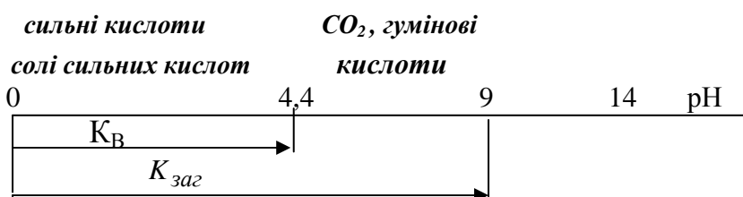
Рис. 3.1. Види кислотності води.
