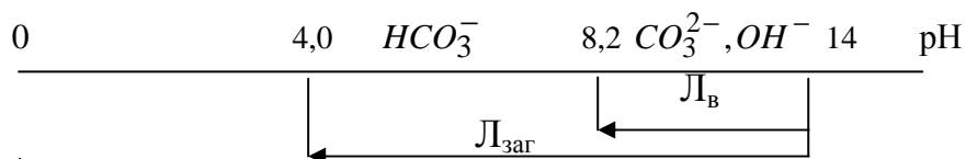
Рис. 3.2. Види лужності води
