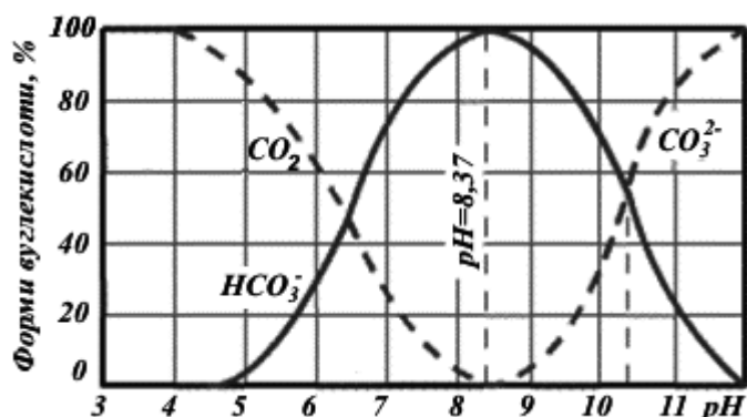
Рис. 3.3. Залежність відсоткового вмісту форм вуглекислоти від рН води.
