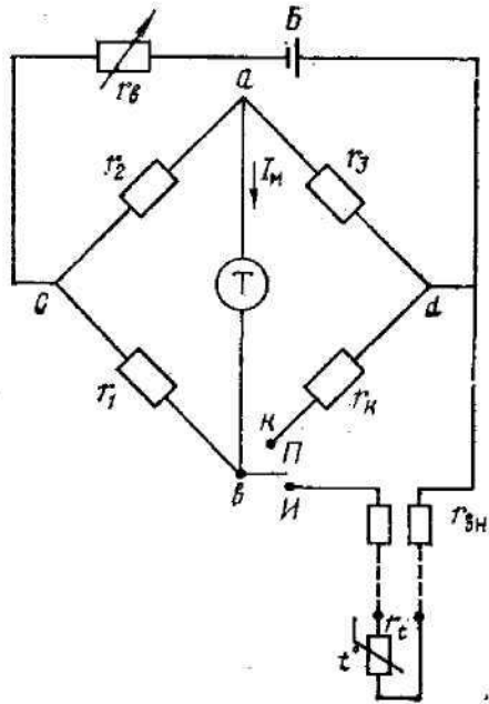
Рис.6.4 - Принципова схема неврівноваженого моста
