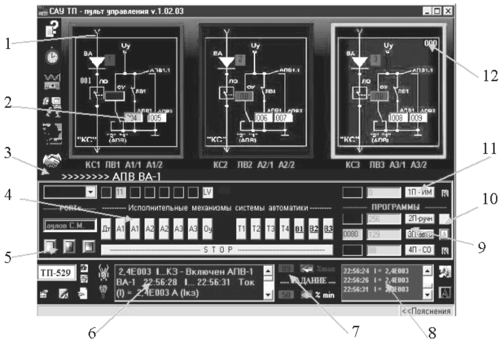
Рис. 10.3 - Интерфейс програми керування ТО:
