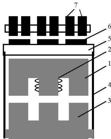
Рис.7.4 - Прямоходовий виконавчий елемент
