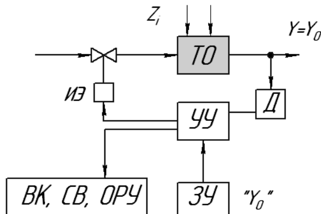
Рис. 2.1 – Блок-схема САР за відхиленням.
