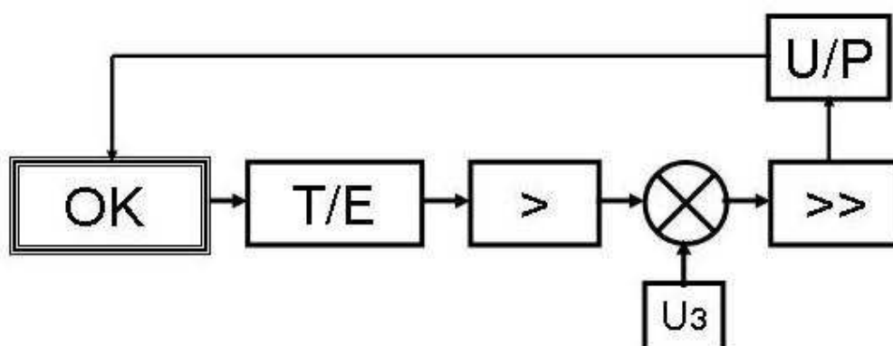
Рис.5.3 - Структурна схема системи автоматики: OK - об'єкт керування; T/E - датчик - перетворювач (параметр - е.р.с.); > - підсилювач напруги; >> - підсилювач потужності; ⊗ - елемент порівняння (суматор); Uз - задатчик; U/P - виконавський елемент (електричний сигнал - механічна дія).
