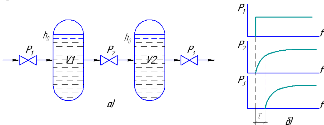
Рис.3.5 – Приклад інерційного об'єкта.
