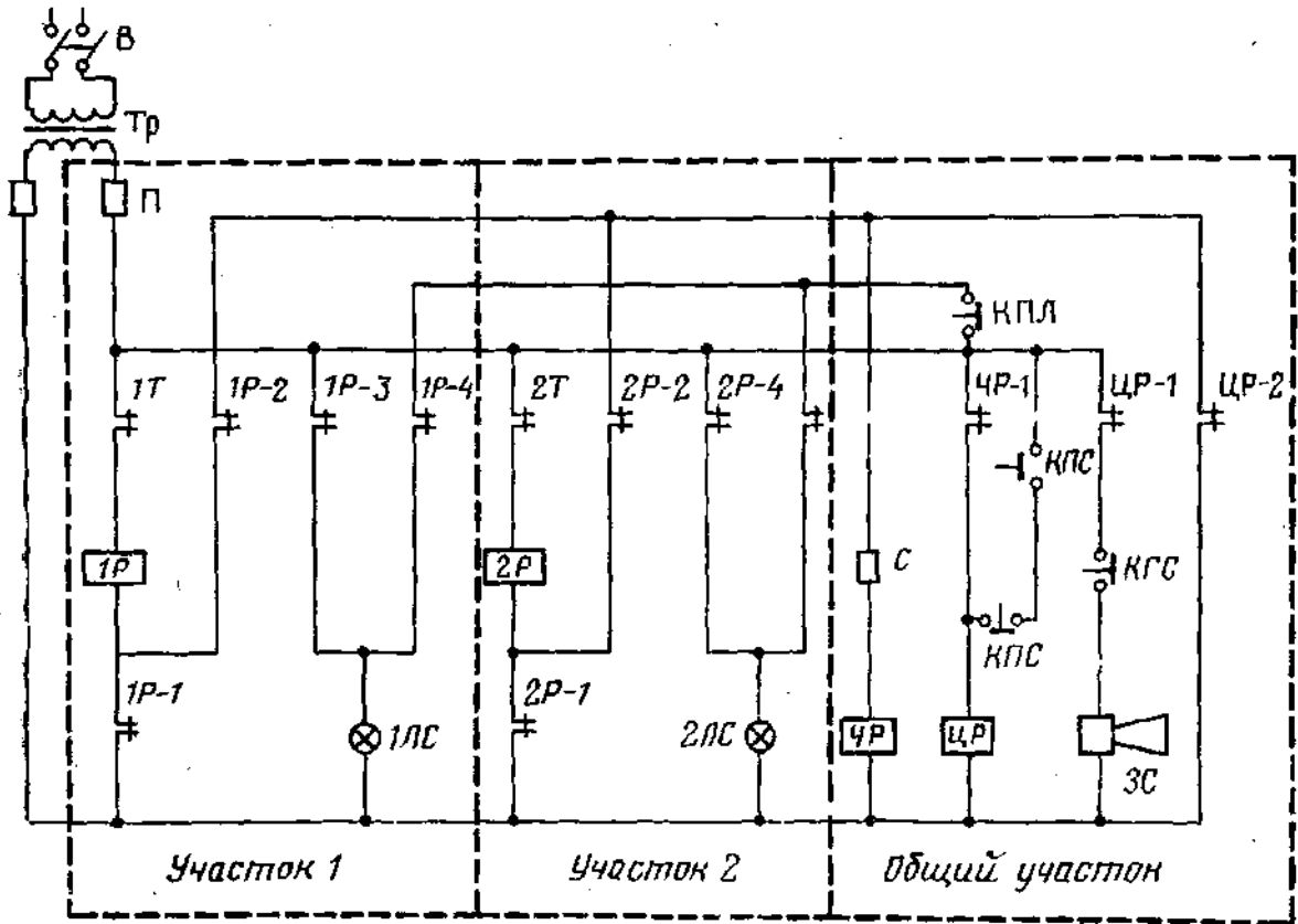
Рис.8.1 - Приклад реальної схеми технологічної сигналізації.
