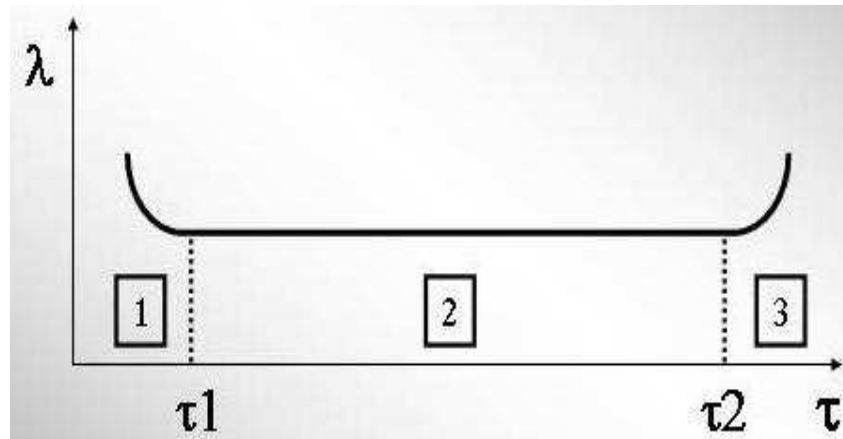
Рис.11.1 – Графік зміни інтенсивності потоку відмов системи
