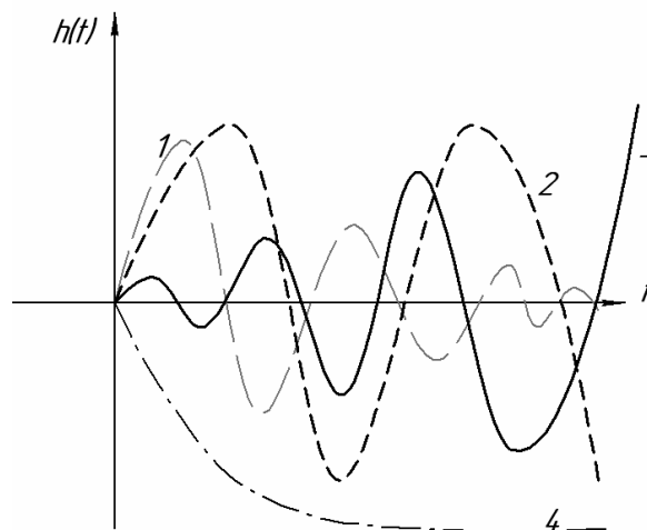
Рис.2.10 - Часові характеристики коливальної ланки:
