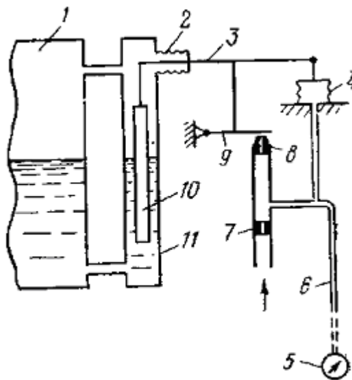
Рис.6.8 - Схема буйкового рівнеміра: 1 - об'єкт контролю; 2 - пружний елемент; 3 - важіль; 4 - сільфон; 5 - вторинний прилад; 6 - сполучна лінія; 7 - дросель постійного перетину; 8 - сопло; 9 - заслінка; 10 - буйок; 11 - камера.
