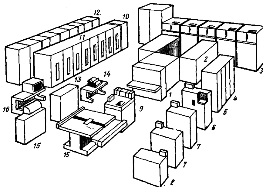
Рис.9.3 - Варіант компонування МПЗА:
