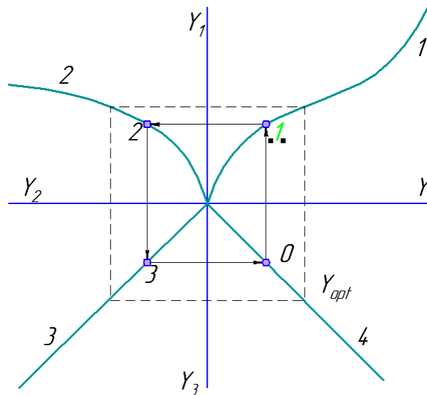
Рис.4.5 - Взаємозв'язок статичних характеристик складного ТО
