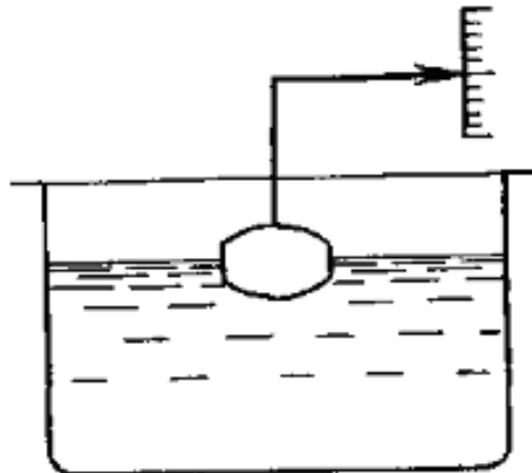
Рис.6.6 - Схема рівнеміра - поплавця.
