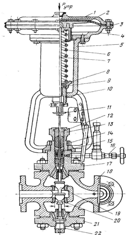
Рис.7.2 - Загальний вигляд двох сідельного регулюючого клапана з пневмоприводом: 1, 4 - кришки головки; 2 - жорсткий центр; 3 - мембрана; 5 - корпус виконавчого механізму; 6 - пружина; 7 - шток; 8 - кільця; 9 - упорний підшипник; 10, 15 - втулки; 11 - покажчик положення плунжера; 12 - ґрундбуksа; 13 - накидна гайка; 14 - сполучна гайка; 16 - лубрика-гор; 17, 18, 21 - фланці; 19 - плунжер; 20 - сідло; 22 - зливна пробка.
