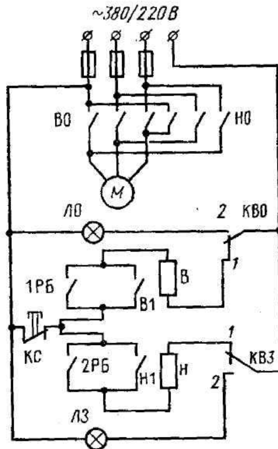
Рис.7.1 - Приклад реальної електричної схеми включення багатообертового виконавчого механізму
