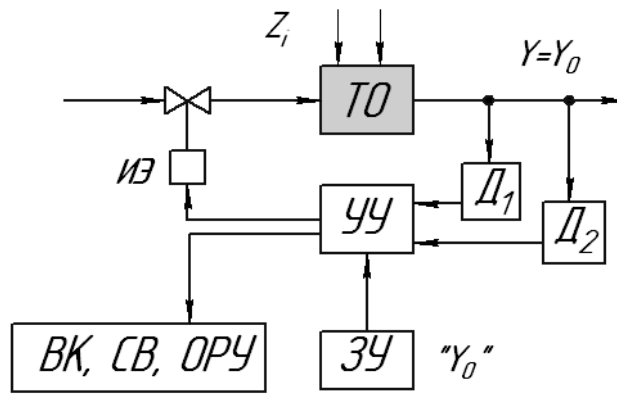
Рис.2.3 – Блок-схема САР комбінована.
