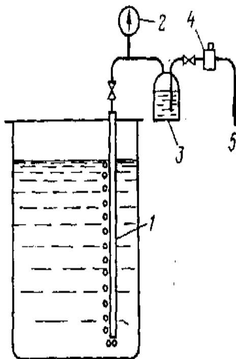
Рис.6.9 - Схема п'езометричного рівнеміра:
