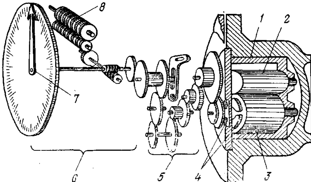
Рис.6.11 - Кінематична схема лічильника з овальними шестернями: 1 - вимірювальна камера; 2, 3 - овальні шестерні; 4- магнітна муфта; 5 - редуктор; 6 - рахунковий механізм; 7 - стрілка; 8 - роликівий рахунковий показчик.
