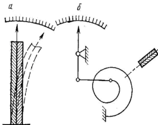
Рис. 6.1 - Схеми біметалічних термометрів: а - з плоским елементом; б - зі спіральним елементом.
