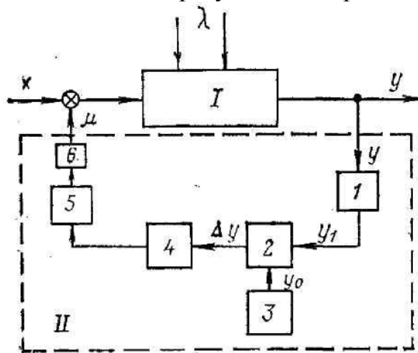
Рис. 5.1 - Структурна схема регулятора: I - об'єкт регулювання; II - регулятор; 1 - датчик; 2 - пристрій порівняння; 3 - задаючий пристрій; 4 - пристрій регулювання; 5 - виконавчий механізм; 6 - регулюючий орган.
