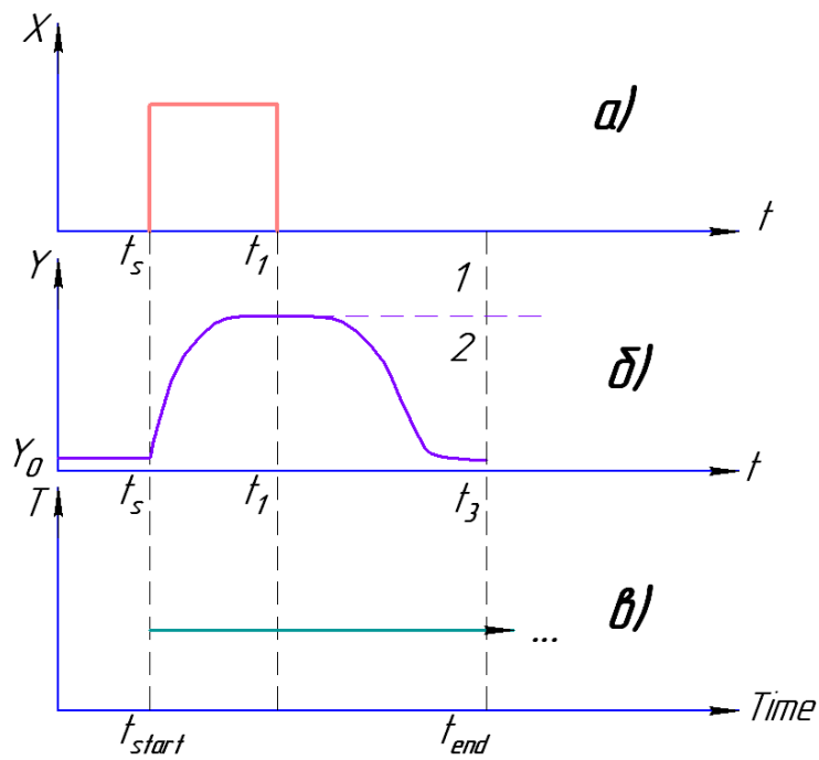
Рис.3.3 - Експериментальне отримання часової характеристики ТО: a - збурююча дія; б - часова характеристика, в - робота таймера пристрою керування ТО.
