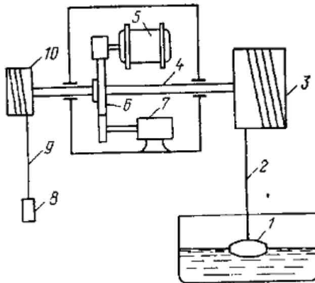
Рис.6.7 - Схема рівнеміра поплавця з сельсином: 1 - поплавець; 2, 9 - троси; 3, 10 - барабани; 4 - вісь; 5 - сельсин-датчик; 6 - зубчасте колесо; 7 - лічильник; 8 - противага.
