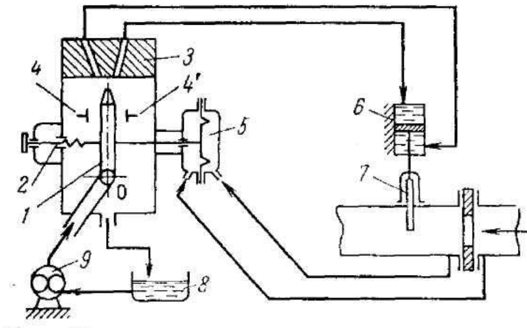
Рис.5.2 - Принципова схема гідравлічного I -регулятора:
