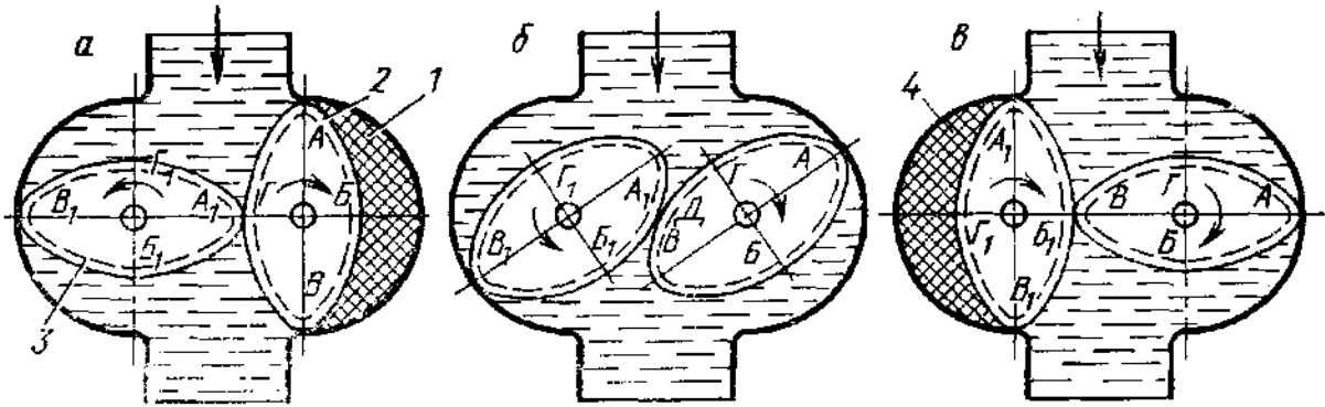
Рис.6.10 - Схема об'ємного рідинного лічильника з овальними шестернями: a - перше початкове положення; б - проміжне положення; в - друге початкове положення; 1 - об'єкт, що витісняється; 2, 3 - овальні шестерні; пунктиром показано зубчасте зачеплення.
