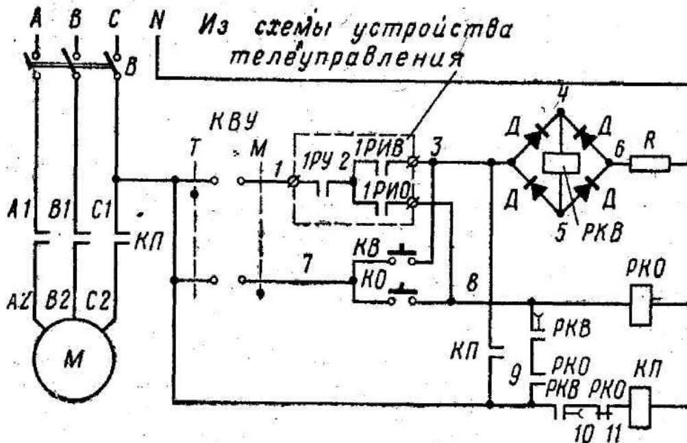
Рис.10.4 - Фрагмент реальної принципової електричної схеми телекерування і місцевого керування асинхронним короткозамкнутим електродвигуном
