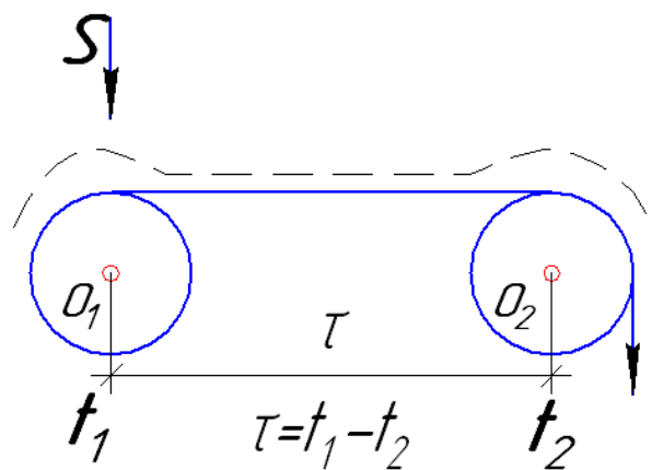
Рис. 3.6 – Приклад транспортного запізнювання
