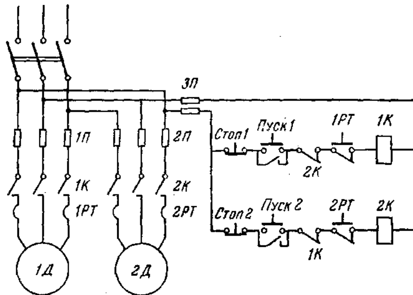
Рис.8.2 - Схема блокування.
