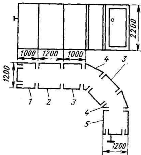
Рис.10.2 - Приклад поєднання щитів (фасад і план) для створення багатошафового Г-подібного щита:
