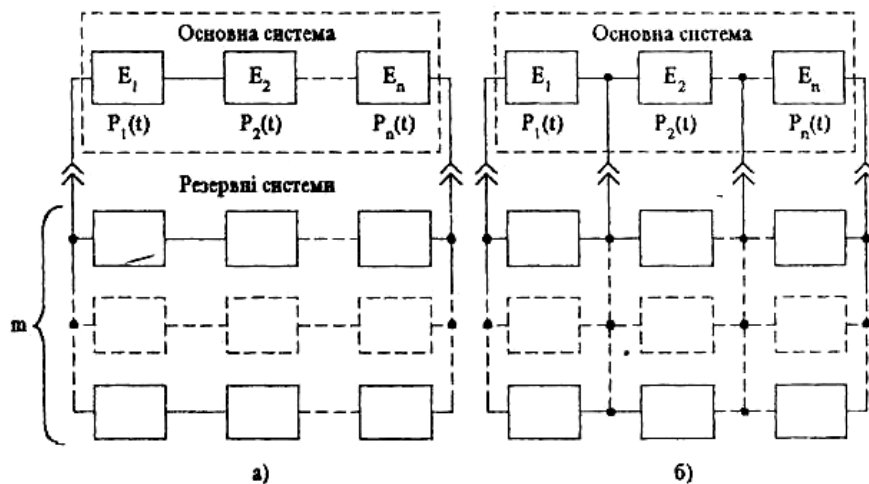
Рис. 11.2 - Схеми структурного резервування: а) загальне; б) поелементне
