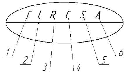
Рис.1.1 - Позначення засобів автоматики на функціональних схемах
