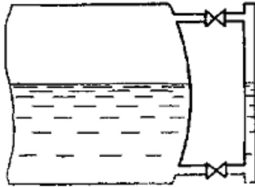
Рис.6.5 - Схема установки з водомірним склом.
