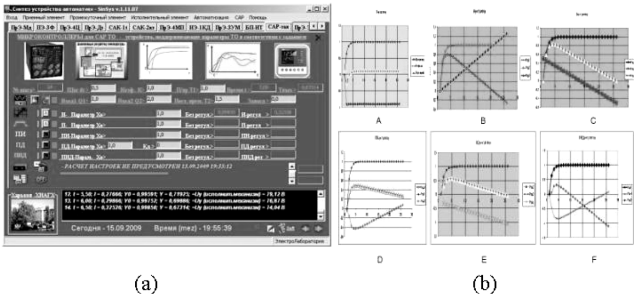
Рис.5.4 - Інтерфейс віртуального стенда (а) і графіки перехідних процесів компонентів САР (b): А - П-регулятор; В - І-регулятор; С - Д-регулятор; D - ІІ-регулятор; E - ПД-регулятор; F - ПІД-регулятор.
