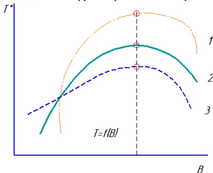
Рис.4.1 - Приклад багатоконтурної системи оптимізації експлуатації ДВЗ при різних режимах: 1 - САР витрати повітря; 2 - САР витрати палива; 3 - САР швидкості руху.
