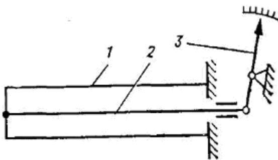
Рис.6.2 - Схема дилатометричного термометра: 1 - трубка; 2 - стрижень; 3 - пристрій для відліку свідчень.
