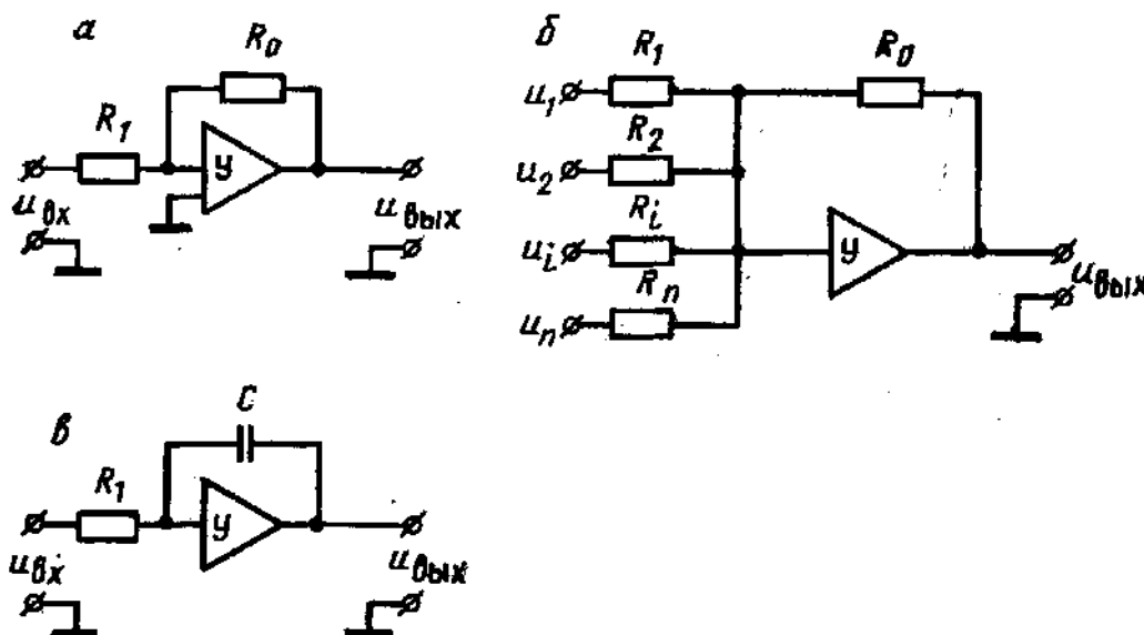
Рис.9.1 - Схеми включення операційних підсилювачів:
