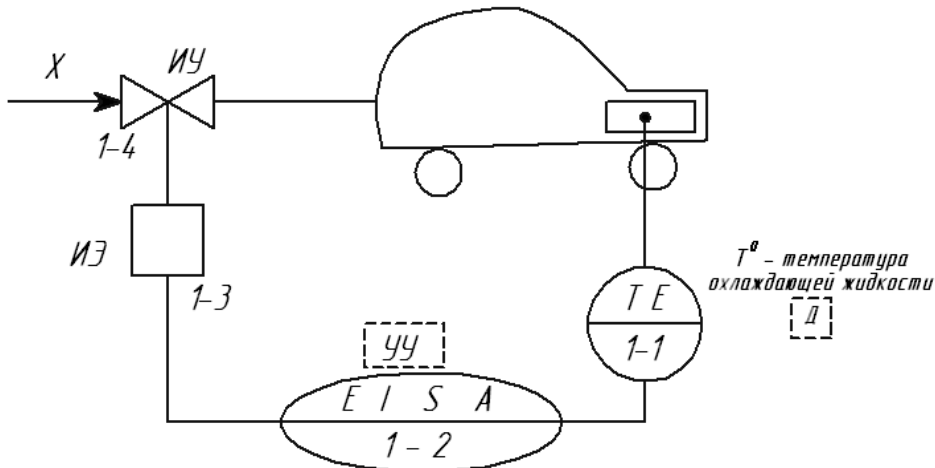
Рис.1.2 - Приклад функціональної схеми
