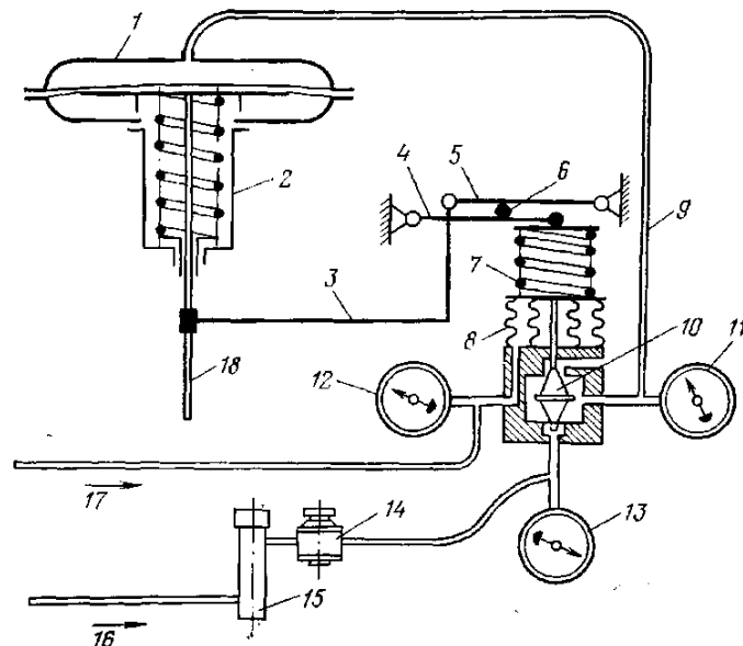
Рис.7.3 - Принципова схема позиційного реле: 1 - головка виконавчого механізму; 2 - виконавчий механізм; 3-5 - важелі; 6 - рухомий шарнір; 7 - пружина; 8 - сифони; 9 - трубка; 10 - клапан; 11-13 - манометри; 14 - редуктор; 15 - фільтр; 16 - повітря від компресора; 17 - повітря від регулятора; 18 - шток.
