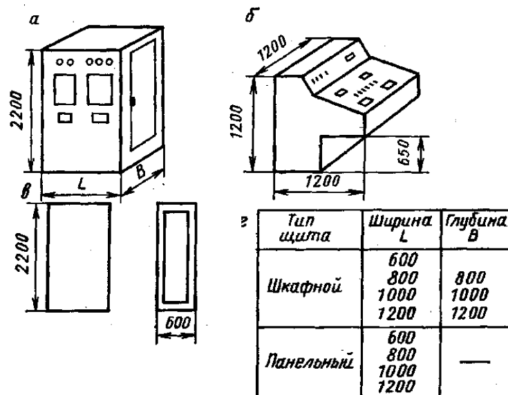
Рис.10.1 - Загальні вигляди шафового щита (а), пульти (б), розміри панельного щита (в) і розміри рекомендованих щитів (г).
