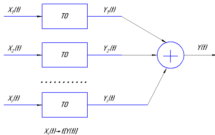
Рис.3.4 – Принцип суперпозиції
