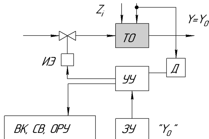
Рис.2.2 – Блок-схема за збуренням.
