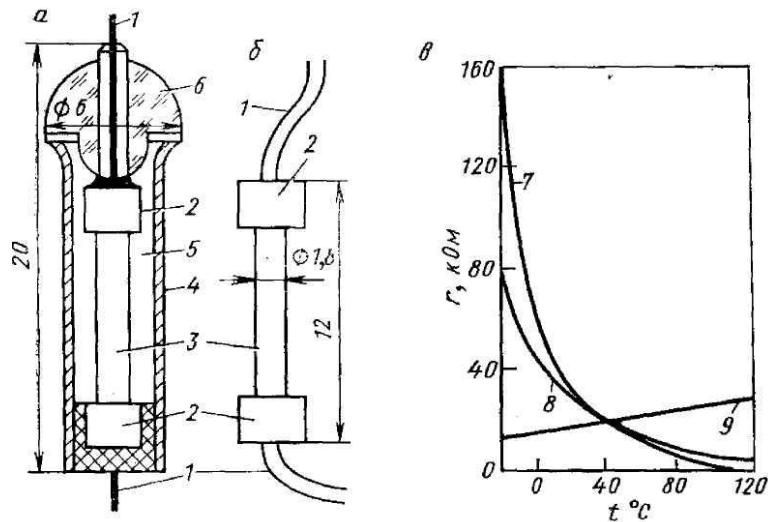
Рис. 6.3 - Загальні види герметизованого (а) і не захищеного (б) терморезисторів і їх температурна характеристика (в):
