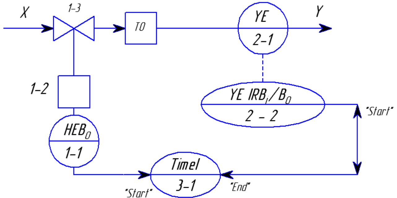
Рис.3.2 – Функціональна схема з експериментального стенда для вивчення ТО
