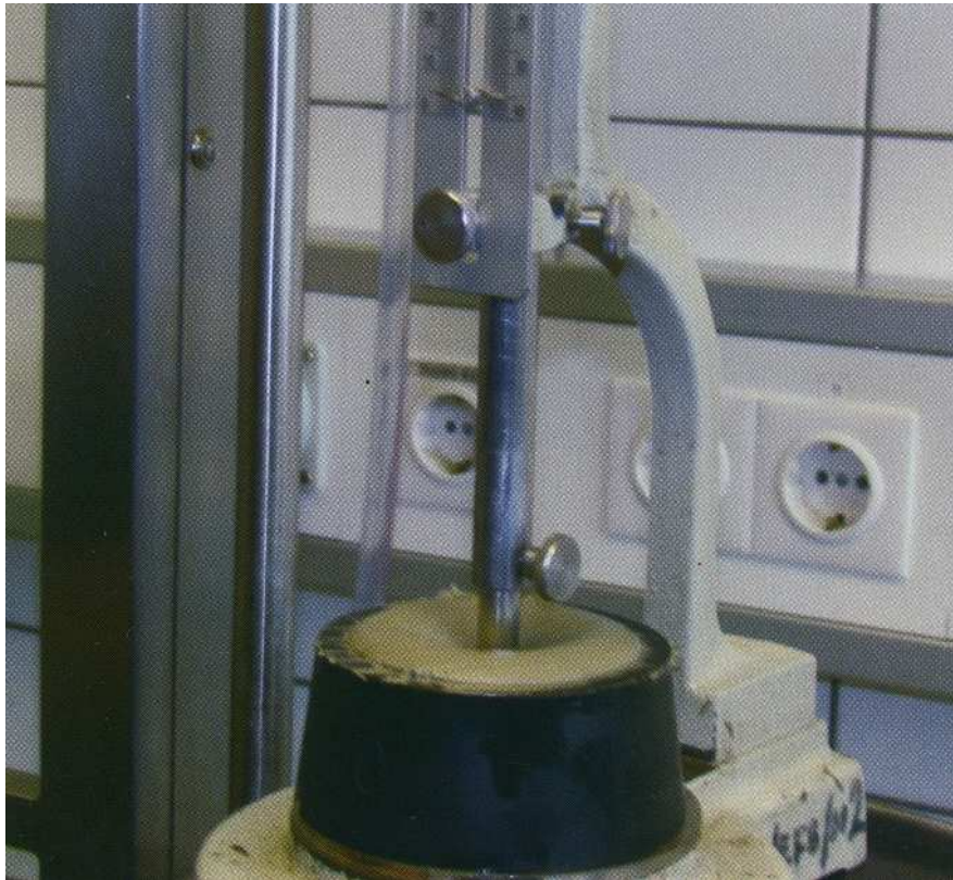
Рис. 3 - Визначення водопотреби цементного тіста
